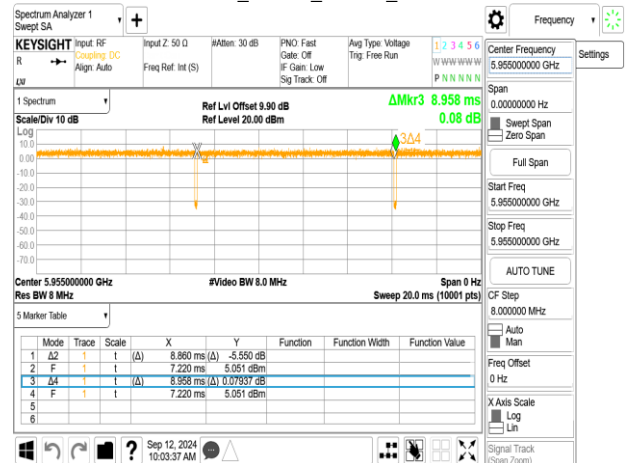
802.11be_20MHz_ChainA_5955MHz_106+26_MRU1
