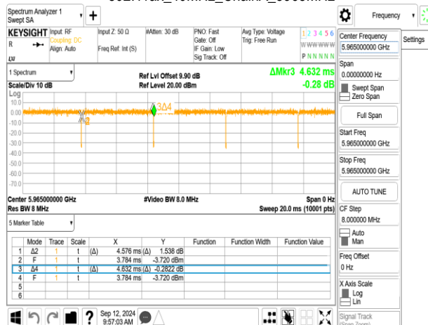
802.11ax 40MHz ChainA 5965MHz RU242 61
