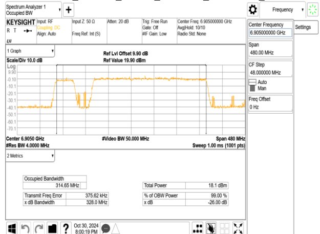
802.11be_320MHz_ChainB_6905MHz_3x996+484_MRU2
