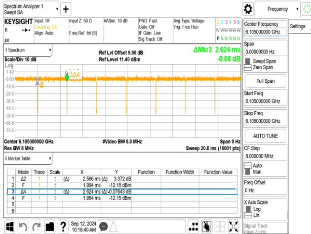
802.11be_320MHz_ChainA_6105MHz_2996+484 MRU2
