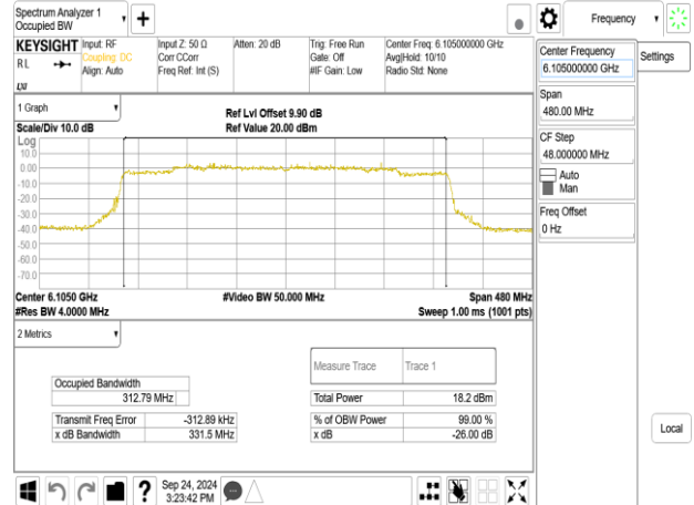
802.11be_320MHz_ChainB_6105MHz_2x996+484_MRUC2
