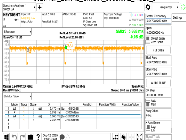
802.11ax 20MHz ChainA 5955MHz RU26 0
