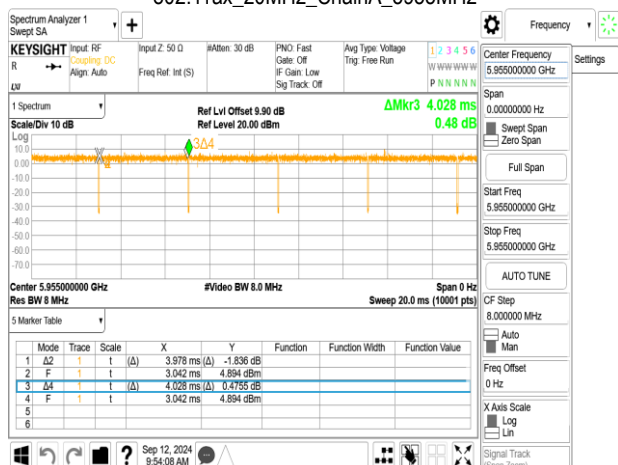
802.11ax 20MHz ChainA 5955MHz RU106 53
