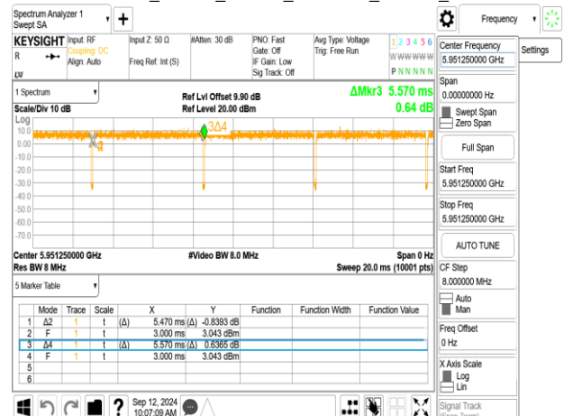
802.11be_20MHz_ChainA_5955MHz_106+26_MRU1
