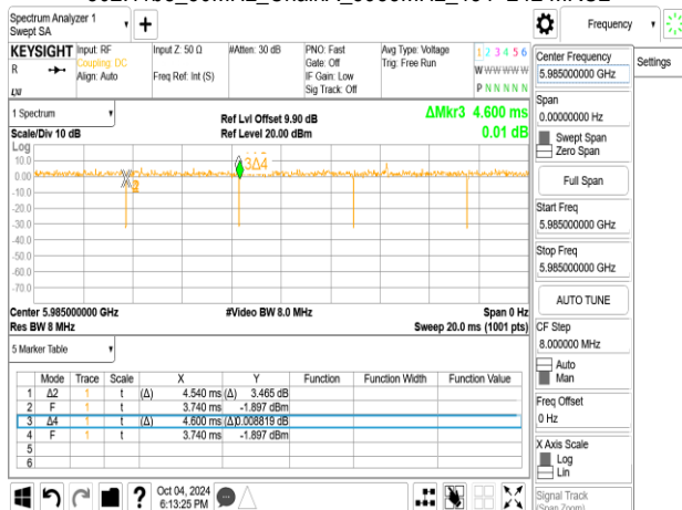
802.11be_80MHz_ChainA_5985MHz_RU484_65
