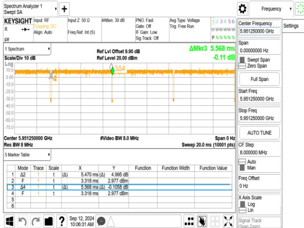
802.11be_20MHz_ChainA_5955MHz_RU106_53
