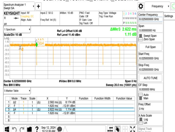
802.11be_160MHz_ChainA_6025MHz_996+484 MRU2
