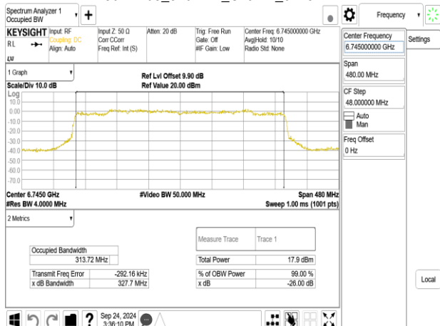
802.11be_320MHz_ChainA_6745MHz
