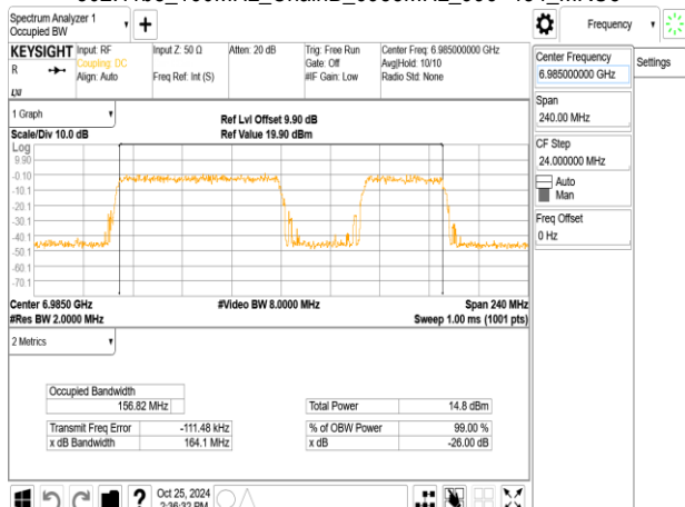
802.11be_160MHz_ChainB_6985MHz_996+484_MRUI4
