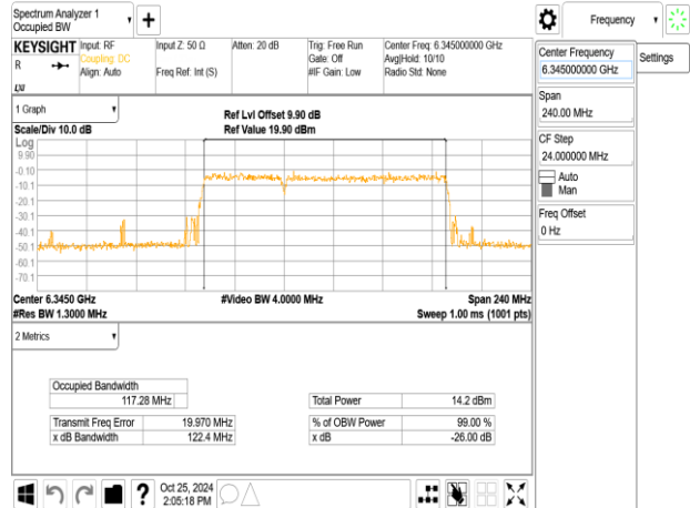
802.11be_160MHz_ChainB_6345MHz_996+484_MRU3
