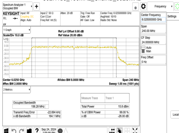
802.11be_160MHz_ChainB_6025MHz_996+484+242_MRU2
