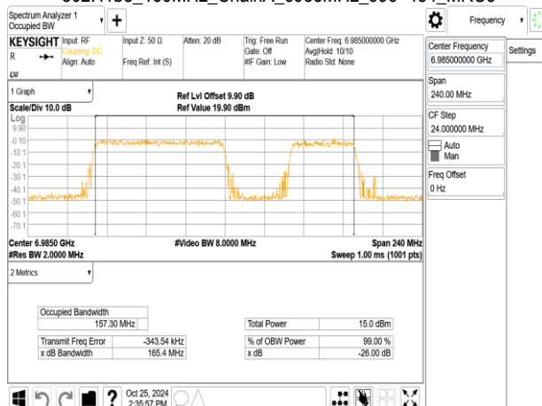
802.11be_160MHz_ChainA_6985MHz_996+484_MRU3
