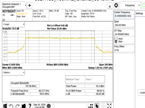
802.11be_160MHz_ChainB_6345MHz
