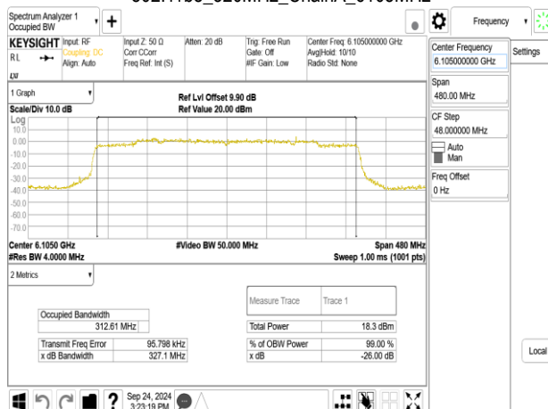
802.11be_320MHz_ChainA_6105MHz_2x996+484_MRUI2
