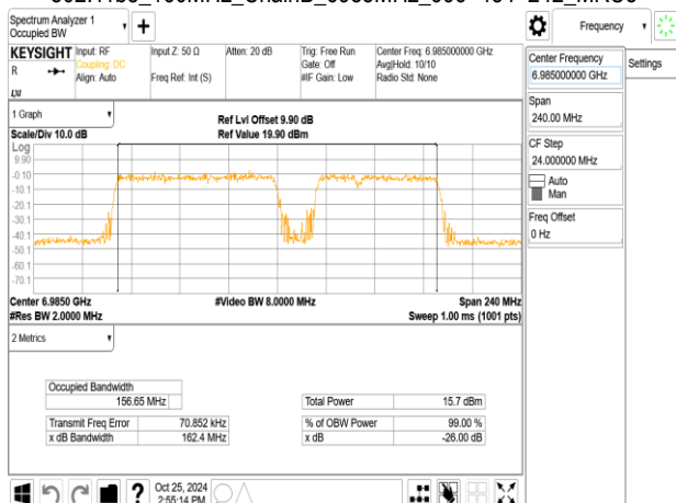
802.11be_160MHz_ChainB_6985MHz_996+484+242_MRU7
