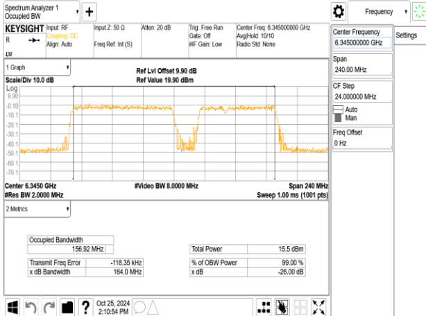
802.11be_160MHz_ChainB_6345MHz_996+484+242_MRU7
