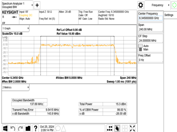
802.11be_160MHz_ChainB_6345MHz_996+484+242_MRU5
