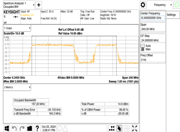
802.11be_160MHz_ChainB_6345MHz_RU996_S67
