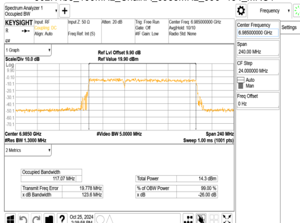
802.11be_160MHz_ChainA_6985MHz_996+484_MRU2
