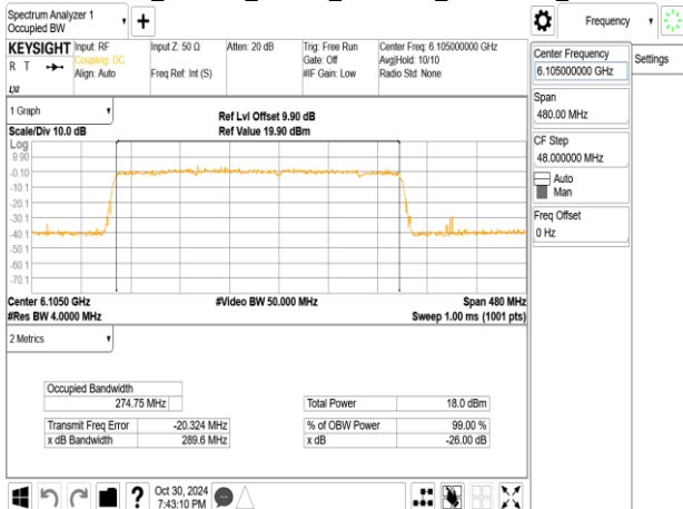
802.11be_320MHz_ChainA_6105MHz_3x996+484_MRUE
