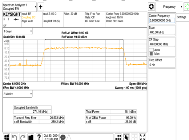
802.11be_320MHz_ChainA_6905MHz_3x996+484_MRU2
