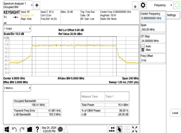
802.11be_160MHz_ChainB_6985MHz_996+484+242_MRU1
