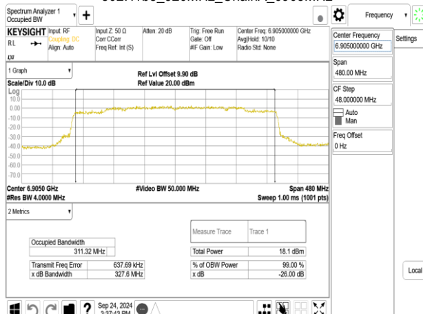
802.11be_320MHz_ChainA_6905MHz_3x996+484_MRU1
