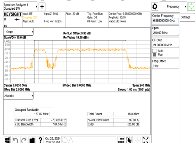
802.11be_160MHz_ChainB_6985MHz_996+484+242_MRU2
