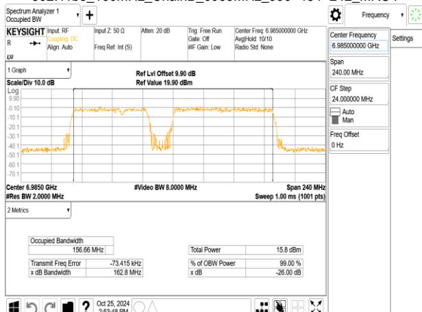
802.11be_160MHz_ChainB_6985MHz_996+484+242_MRU5
