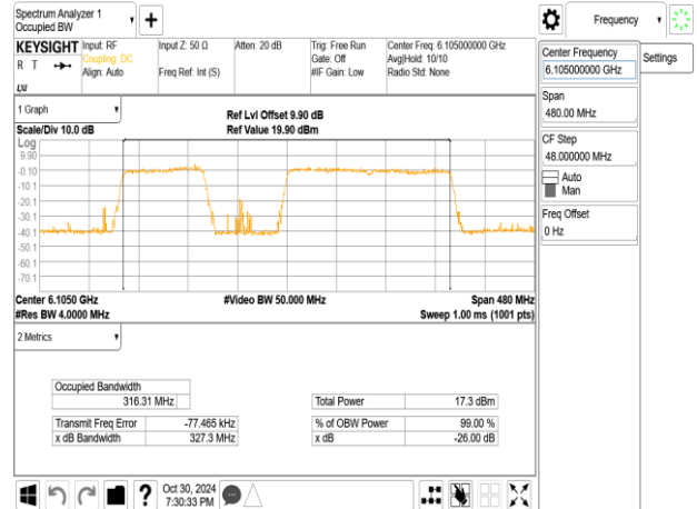
802.11be_320MHz_ChainA_6105MHz_3x996_MRUE
