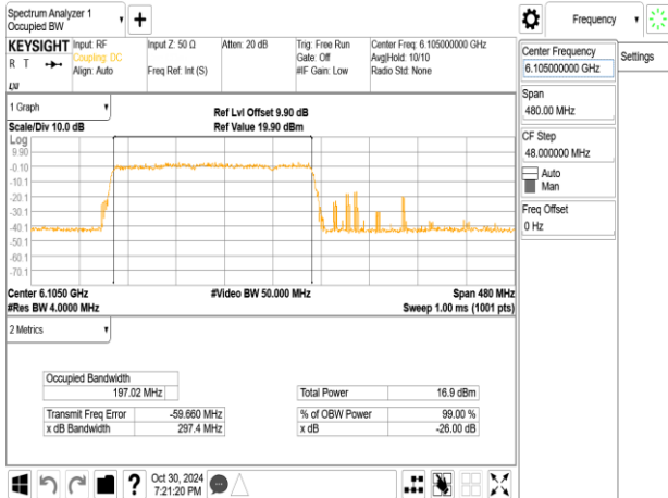
802.11be_320MHz_ChainA_6105MHz_3x996+484_MRUE
