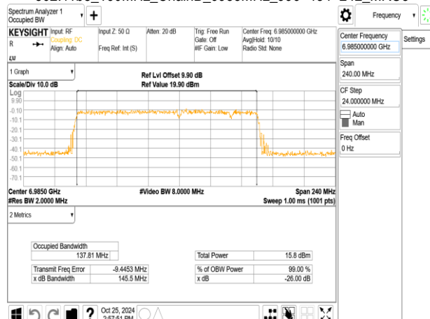
802.11be_160MHz_ChainB_6985MHz_996+484_MRU1
