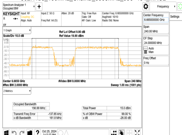
802.11be_160MHz_ChainB_6665MHz_996+484_MRU3
