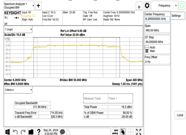
802.11be_320MHz_ChainA_6265MHz
