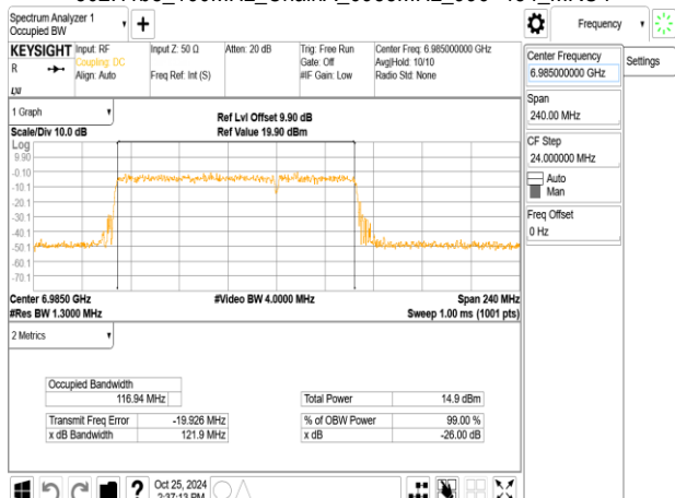
802.11be_160MHz_ChainA_6985MHz_RU996_67
