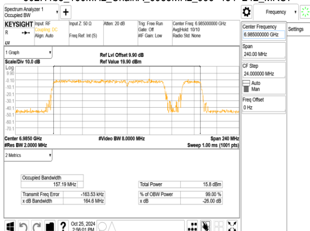
802.11be_160MHz_ChainA_6985MHz_996+484+242_MRU8
