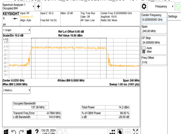
802.11be_160MHz_ChainB_6025MHz_996+484_MRU2
