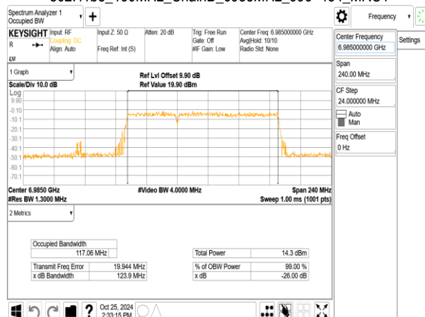
802.11be_160MHz_ChainB_6985MHz_996+484_MRU2
