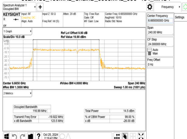
802.11be_160MHz_ChainB_6665MHz_996+484_MRU4
