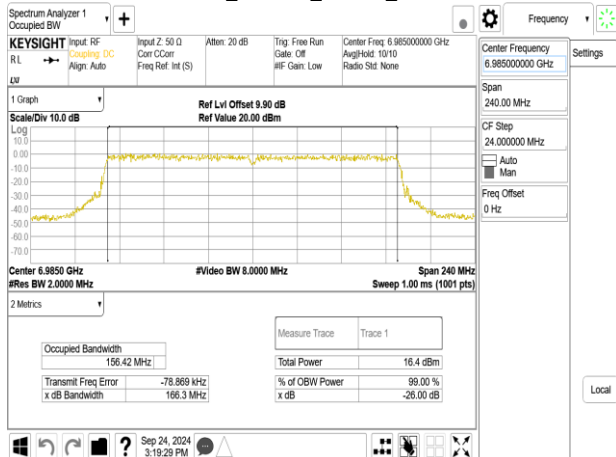
802.11be_160MHz_ChainA_6985MHz
