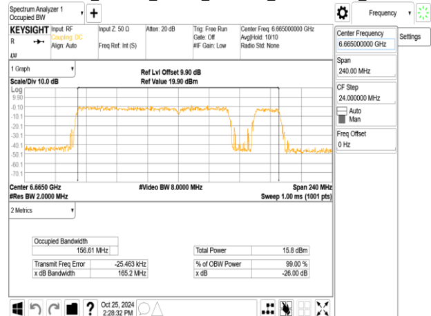
802.11be_160MHz_ChainA_6665MHz_996+484+242_MRU7
