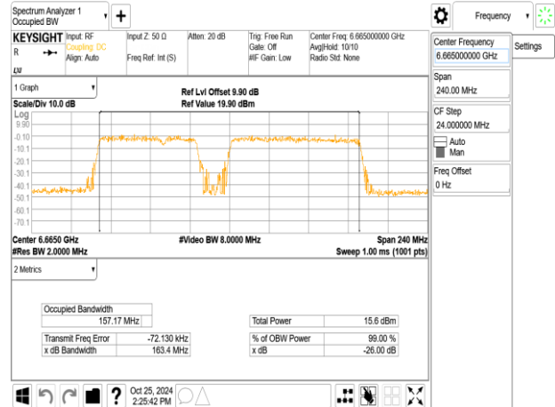
802.11be_160MHz_ChainA_6665MHz_996+484+242_MRU5
