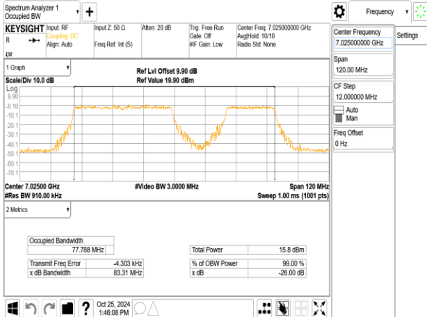
802.11be_80MHz_ChainA_7025MHz_RU484_66
