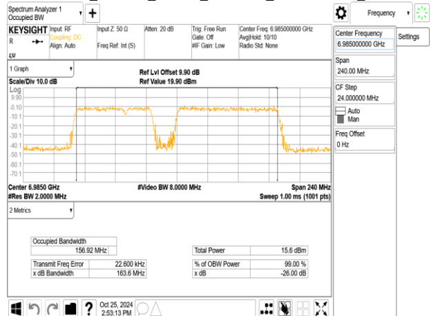
802.11be_160MHz_ChainA_6985MHz_996+484+242_MRU4
