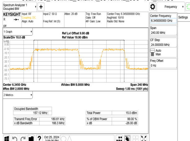
802.11be_160MHz_ChainA_6345MHz_RU996_S67
