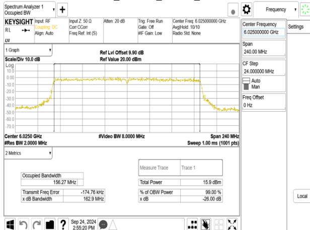
802.11be_160MHz_ChainA_6025MHz
