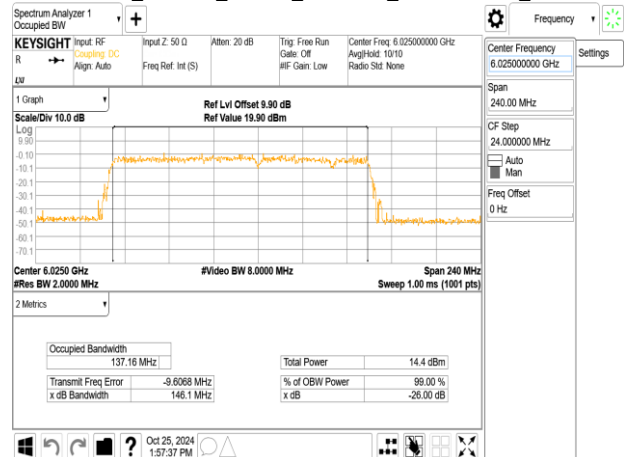
802.11be_160MHz_ChainA_6025MHz_996+484+242_MRU8
