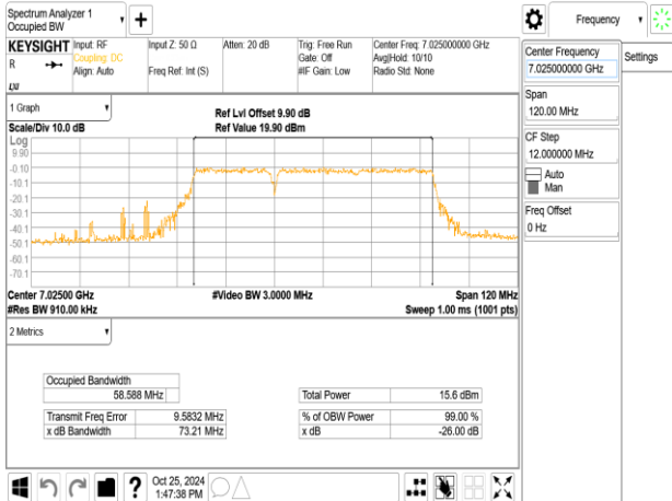
802.11be_80MHz_ChainA_7025MHz_484+242_MRU3
