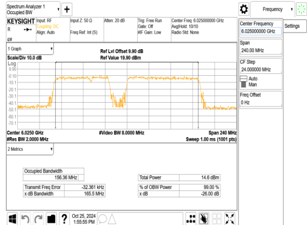
802.11be_160MHz_ChainA_6025MHz_996+484+242_MRU8
