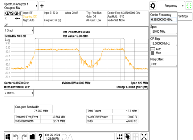
802.11be_80MHz_ChainB_6385MHz_RU484_66
