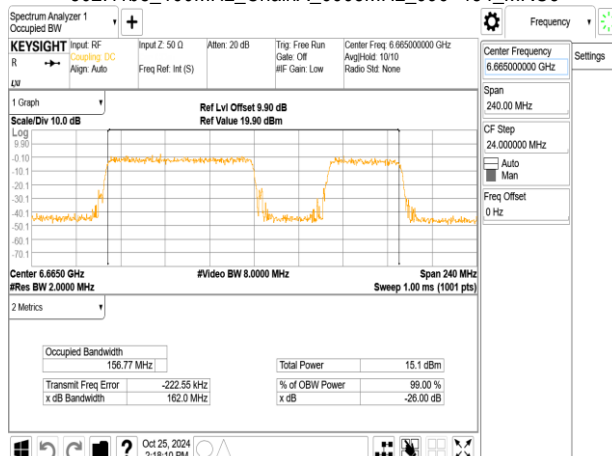
802.11be_160MHz_ChainA_6665MHz_996+484_MRU4
