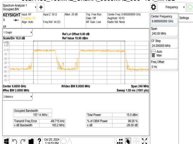
802.11be_160MHz_ChainA_6665MHz_996+484_MRU2
