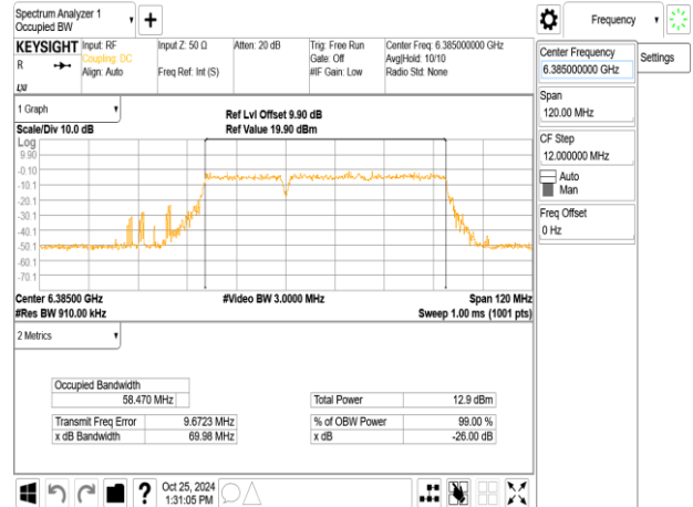
802.11be_80MHz_ChainB_6385MHz_484+242_MRU3
