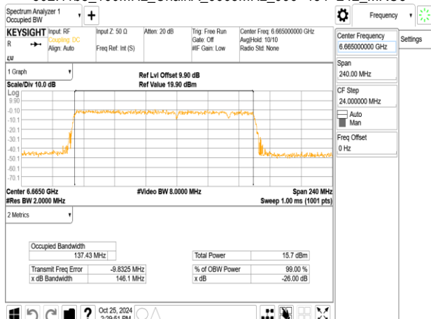
802.11be_160MHz_ChainA_6665MHz_996+484_MRU1
