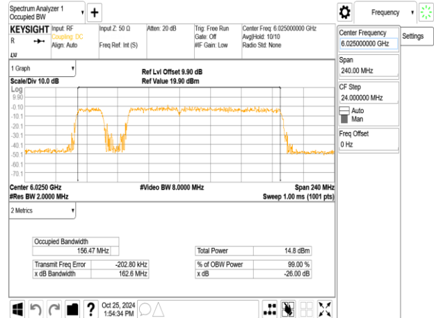
802.11be_160MHz_ChainA_6025MHz_996+484+242_MRU4
