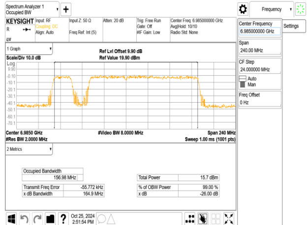
802.11be_160MHz_ChainA_6985MHz_996+484+242_MRU4
