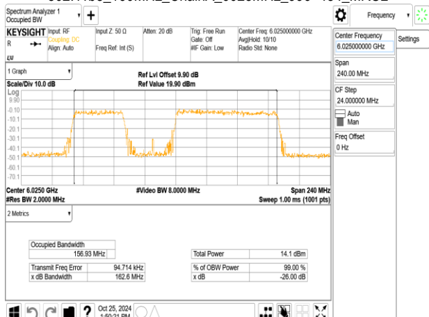
802.11be_160MHz_ChainA_6025MHz_996+484_MRU4
