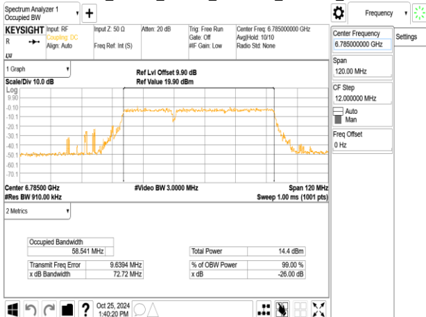
802.11be_80MHz_ChainB_6785MHz_484+242_MRU1
