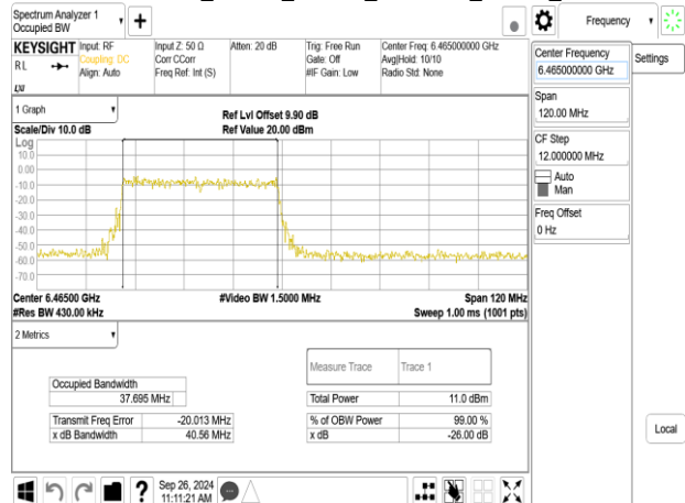
802.11be_80MHz_ChainB_6465MHz_RU484_65
