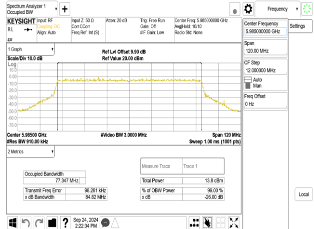
802.11be_80MHz_ChainB_5985MHz_484+242_MRU2
