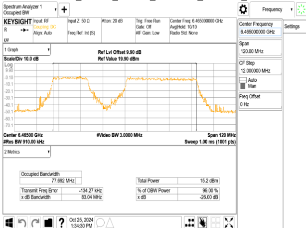
802.11be_80MHz_ChainB_6465MHz_484+242_MRU2
