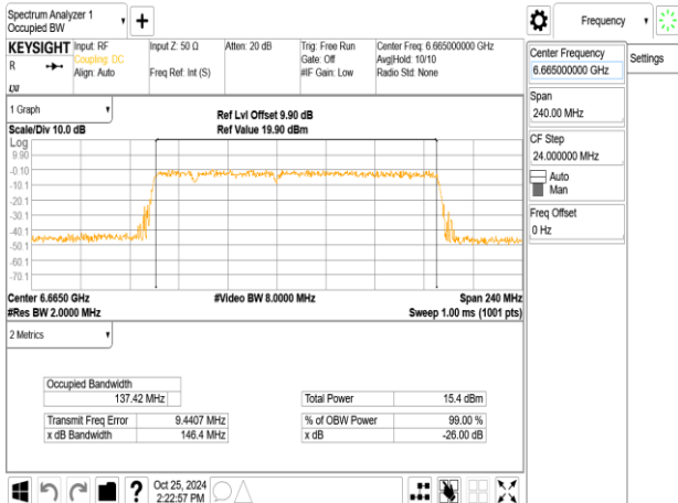
802.11be_160MHz_ChainA_6665MHz_996+484+242_MRU2
