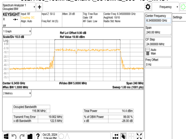
802.11be_160MHz_ChainA_6345MHz_996+484_MRU1
