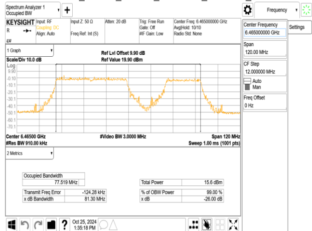
802.11be_80MHz_ChainB_6465MHz_484+242_MRU4
