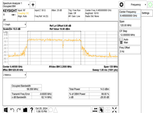
802.11be_80MHz_ChainB_6465MHz_RU484_65
