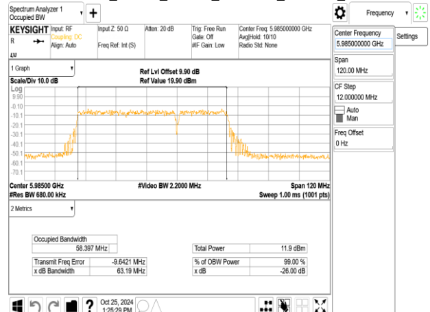
802.11be_80MHz_ChainB_5985MHz_484+242_MRU4
