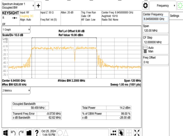
802.11be_80MHz_ChainB_6945MHz_484+242_MRU4
