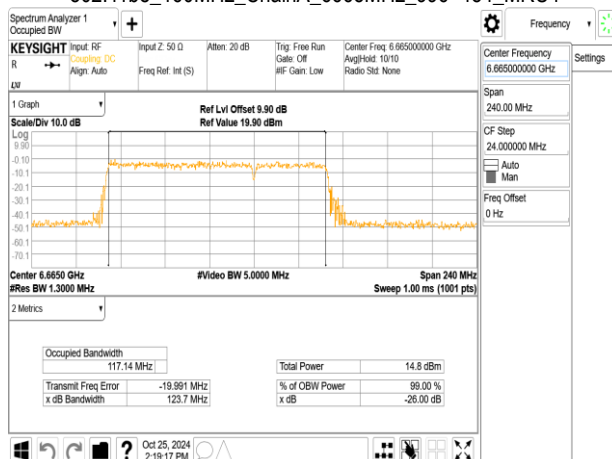
802.11be_160MHz_ChainA_6665MHz_RU996_67
