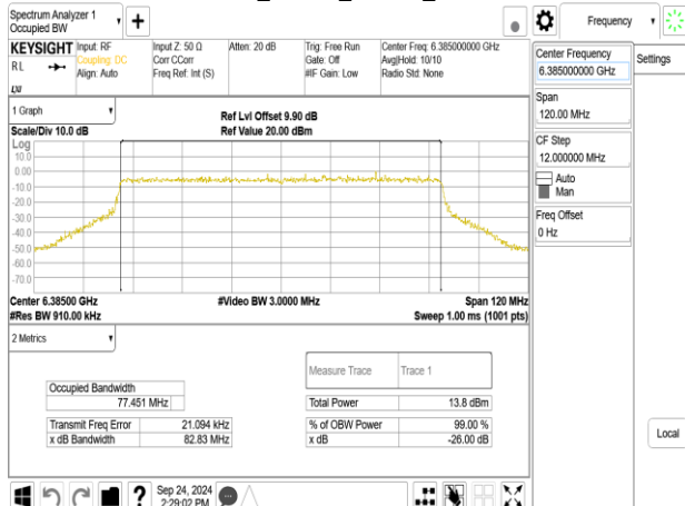
802.11be_80MHz_ChainB_6385MHz
