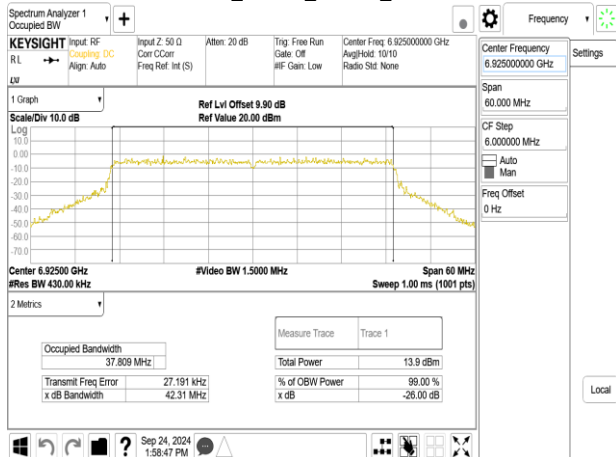
802.11be_40MHz_ChainA_6925MHz
