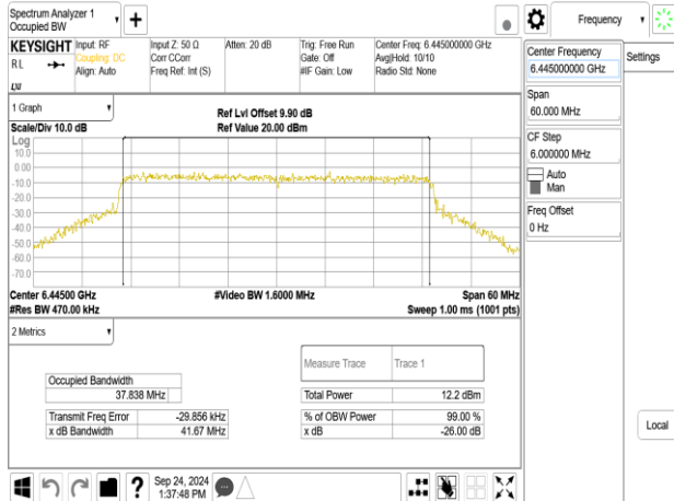
802.11be_40MHz_ChainB_6445MHz_RU242_61
