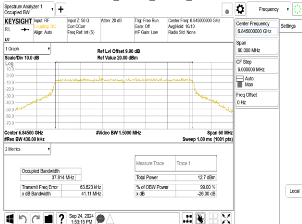
802.11be_40MHz_ChainB_6845MHz
