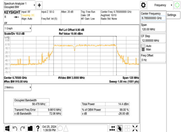
802.11be_80MHz_ChainA_6785MHz_484+242_MRU3
