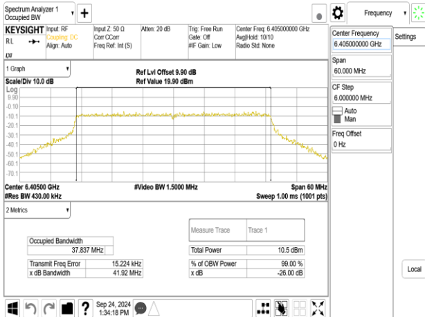
802.11be_40MHz_ChainA_6405MHz_RU242_62
