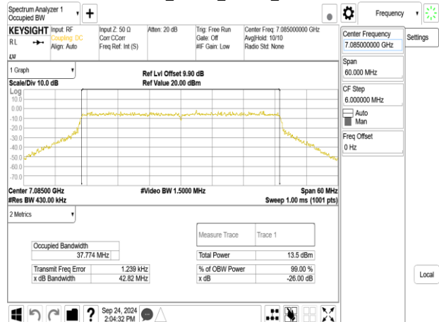
802.11be_40MHz_ChainA_7085MHz
