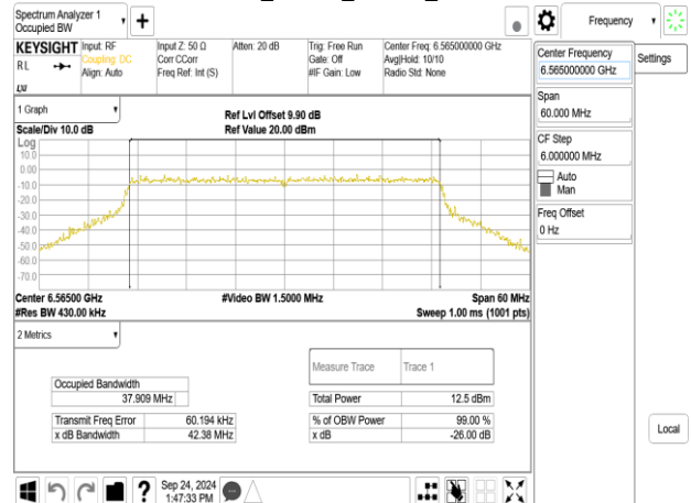
802.11be_40MHz_ChainB_6565MHz
