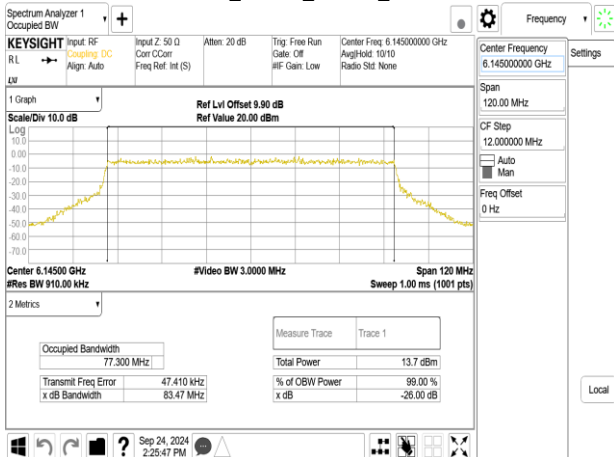
802.11be_80MHz_ChainA_6145MHz
