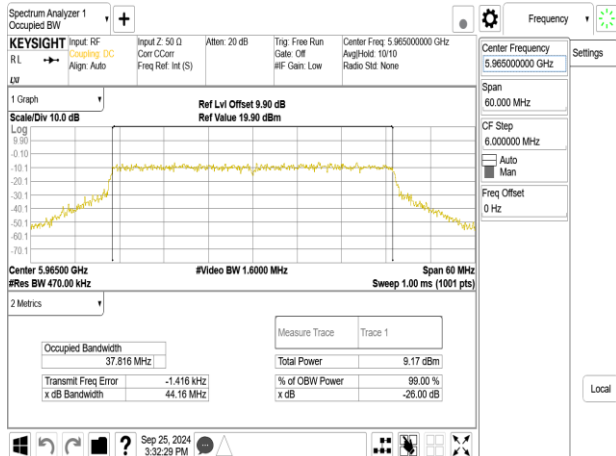
802.11be_40MHz_ChainB_5965MHz_RU242_61
