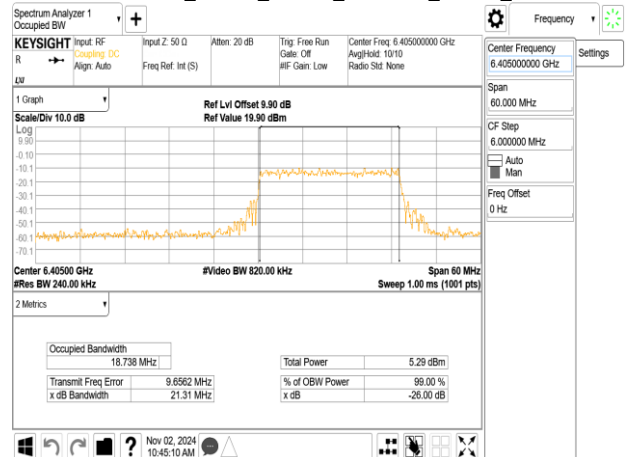
802.11be_40MHz_ChainB_6405MHz_RU242_62
