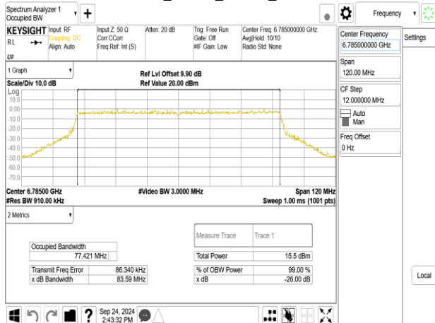
802.11be_80MHz_ChainA_6785MHz
