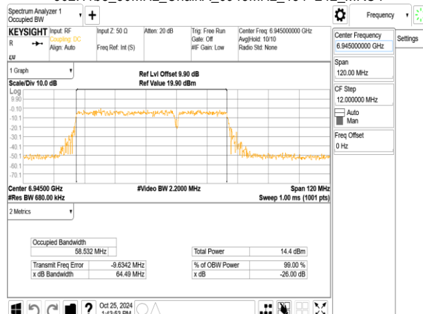
802.11be_80MHz_ChainA_6945MHz_RU484_65
