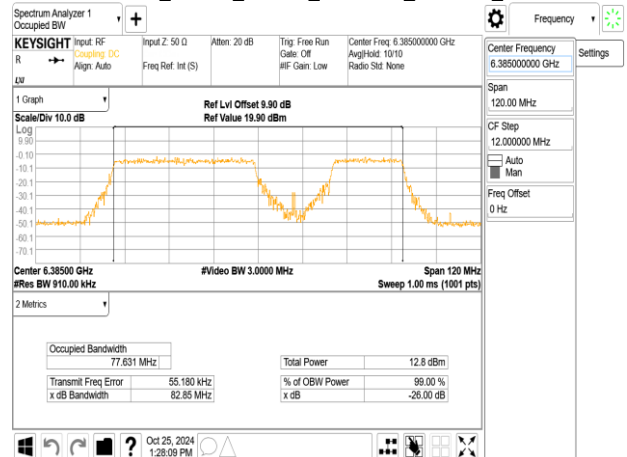
802.11be_80MHz_ChainA_6385MHz_484+242_MRU3
