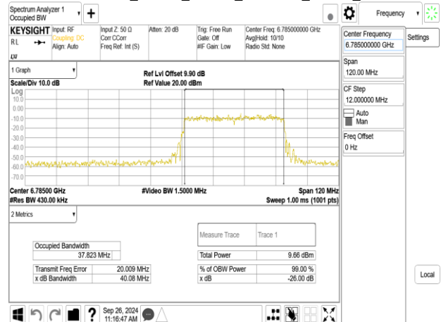
802.11be_80MHz_ChainA_6785MHz_RU484_66
