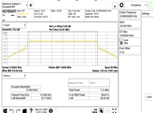
802.11be_40MHz_ChainA_6565MHz
