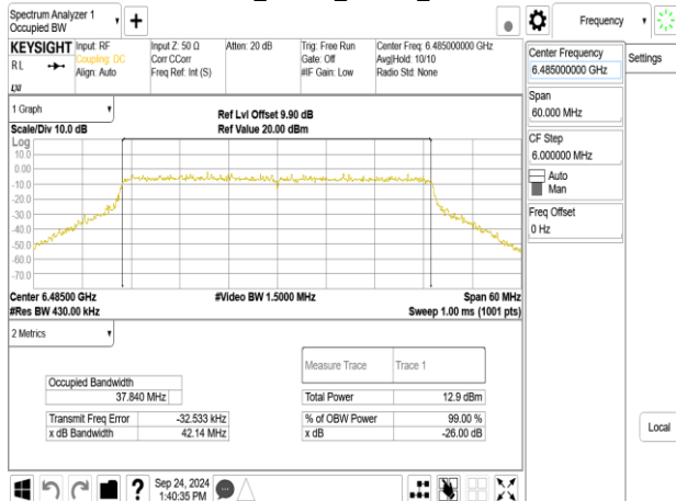
802.11be_40MHz_ChainB_6485MHz
