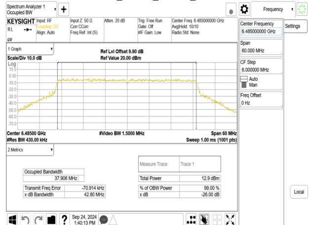
802.11be_40MHz_ChainA_6485MHz
