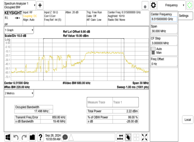
802.11be_20MHz_ChainB_6515MHz_RU26_8
