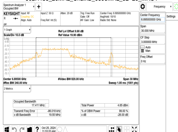
802.11be_20MHz_ChainB_6895MHz_52+26_MRU1
