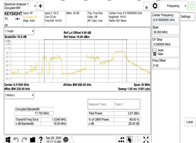
802.11be_20MHz_ChainB_6515MHz_RU26_8
