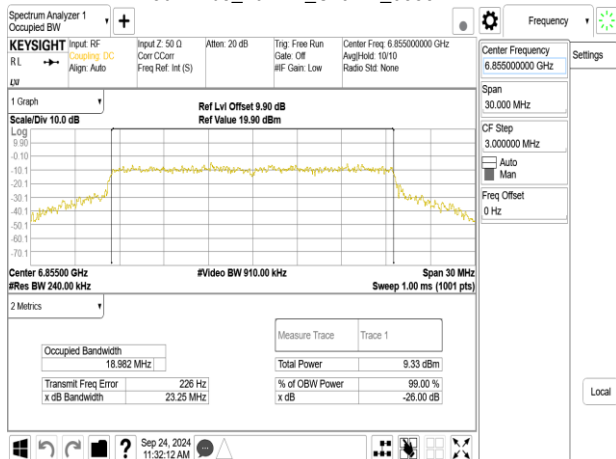
802.11be_20MHz_ChainB_6855MHz
