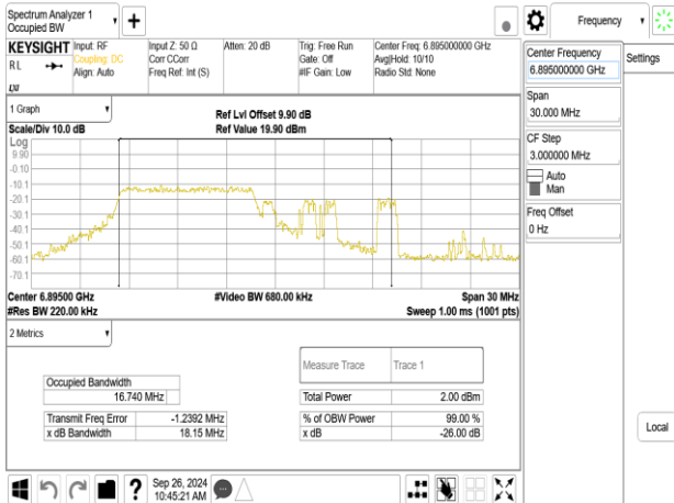
802.11be_20MHz_ChainA_6895MHz_RU26_0
