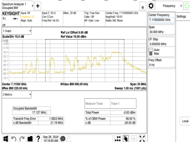
802.11be_20MHz_ChainB_7115MHz_RU26_8
