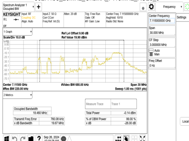
802.11be_20MHz_ChainA_7115MHz_RU52_40
