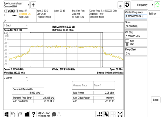
802.11be_20MHz_ChainA_7115MHz
