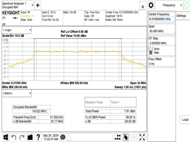
802.11be_20MHz_ChainB_6515MHz_106+26_MRJ2
