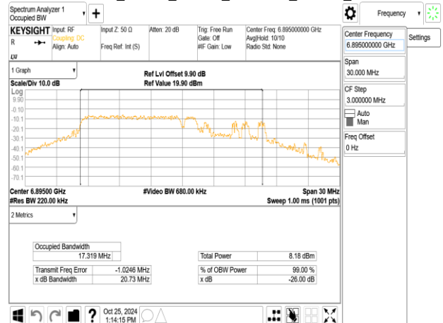
802.11be_20MHz_ChainA_6895MHz_106+26_MRUI
