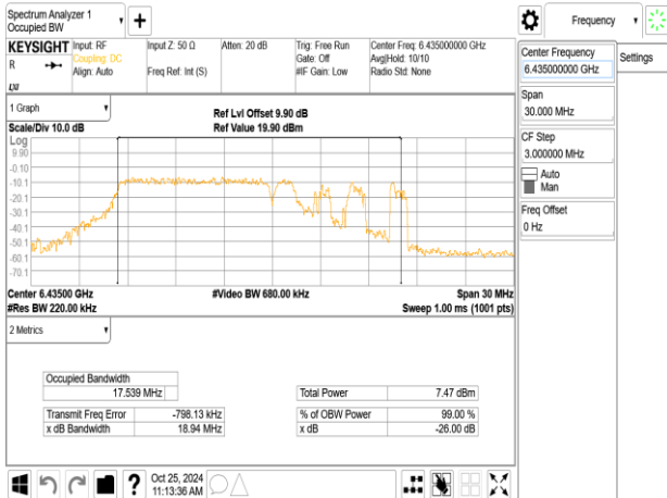
802.11be_20MHz_ChainB_6435MHz_52+26_MRU1
