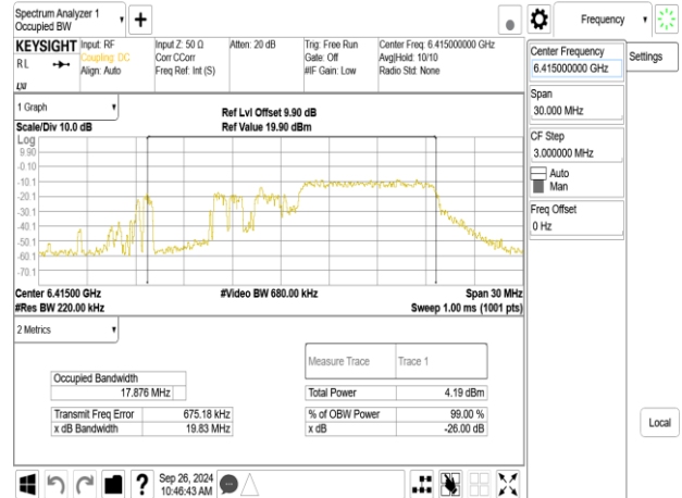
802.11be_20MHz_ChainB_6415MHz_RU26_8
