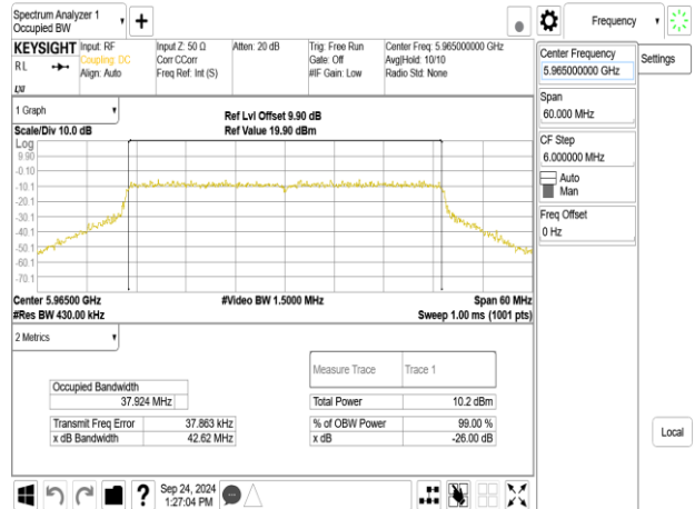
802.11be_40MHz_ChainA_5965MHz_RU242_61
