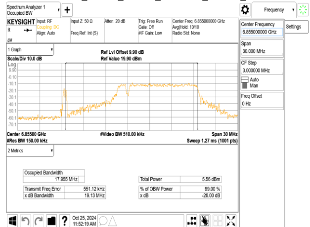
802.11be_20MHz_ChainB_6855MHz_52+26_MRJ3
