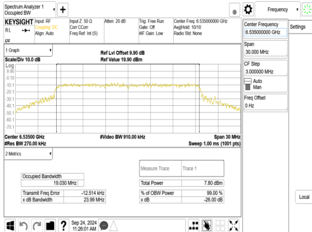
802.11be_20MHz_ChainB_6535MHz_106+26_MRUI
