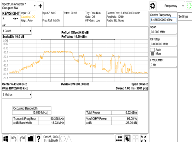
802.11be_20MHz_ChainB_6435MHz_52+26_MRU1
