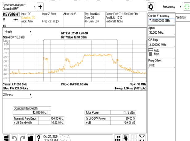
802.11be_20MHz_ChainA_7115MHz_RU106_54
