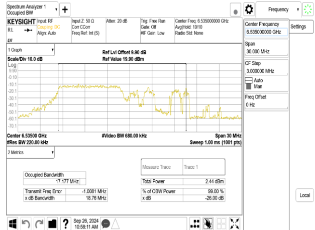
802.11be_20MHz_ChainB_6535MHz_RU26_0
