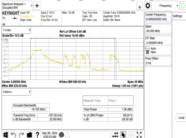
802.11be_20MHz_ChainA_6895MHz_RU26_0
