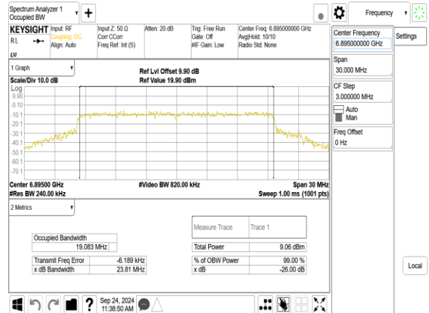
802.11be_20MHz_ChainA_6895MHz_106+26_MRUI
