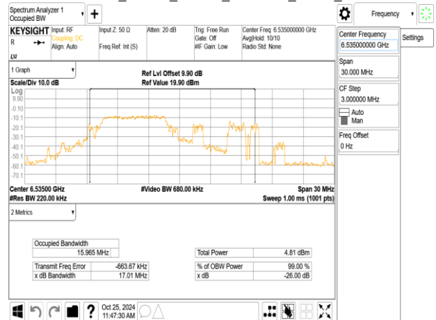
802.11be_20MHz_ChainB_6535MHz_RU106_53
