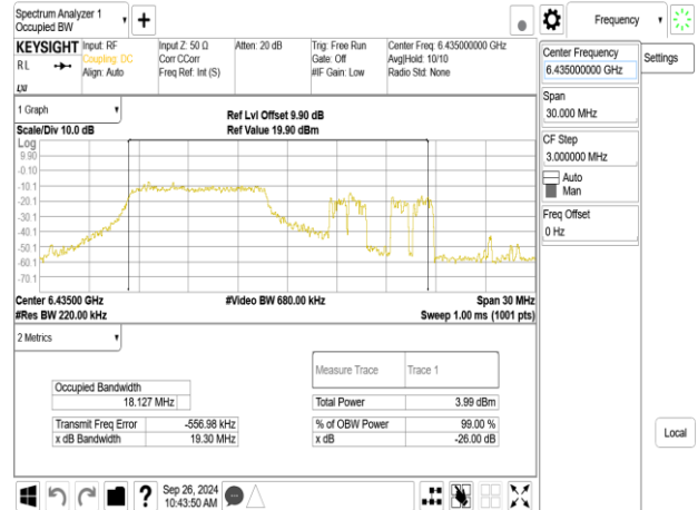
802.11be_20MHz_ChainB_6435MHz_RU26_0
