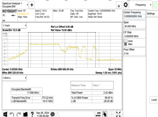
802.11be_20MHz_ChainB_5955MHz_RU106_53
