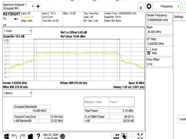
802.11be_20MHz_ChainB_5955MHz
