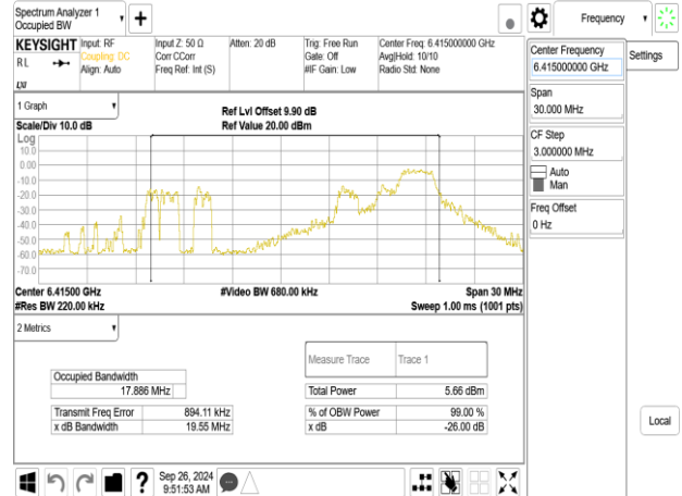
802.11be_20MHz_ChainB_6415MHz_RU52_40
