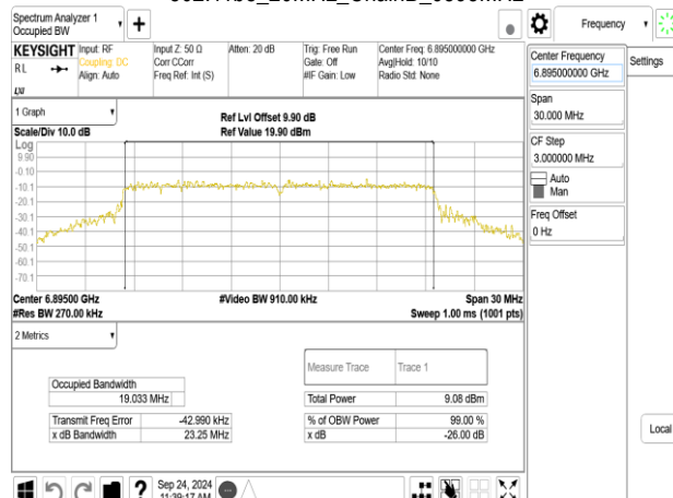
802.11be_20MHz_ChainB_6895MHz_106+26_MRU1
