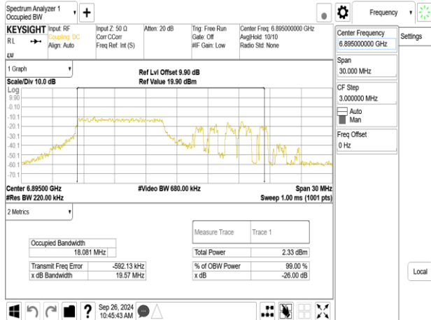
802.11be_20MHz_ChainB_6895MHz_RU26_0
