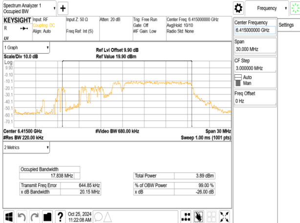
802.11be_20MHz_ChainB_6415MHz_52+26_MRU3
