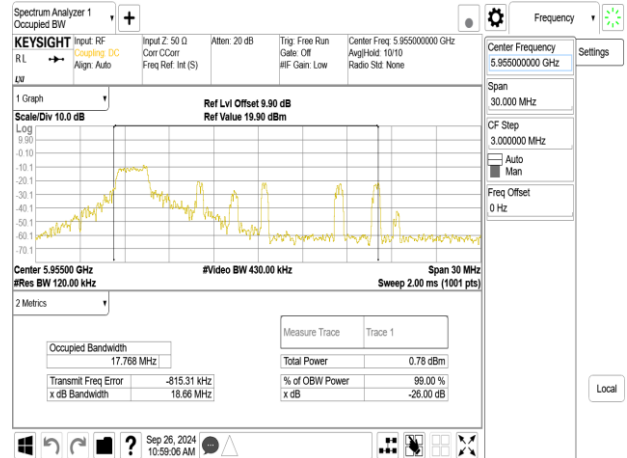
802.11be_20MHz_ChainB_5955MHz_RU52_37
