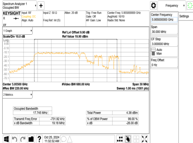
802.11be_20MHz_ChainB_5955MHz_52+26_MRU1
