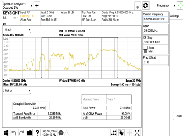
802.11be_20MHz_ChainA_6855MHz_RU52_40
