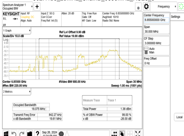
802.11be_20MHz_ChainB_6855MHz_RU52_40
