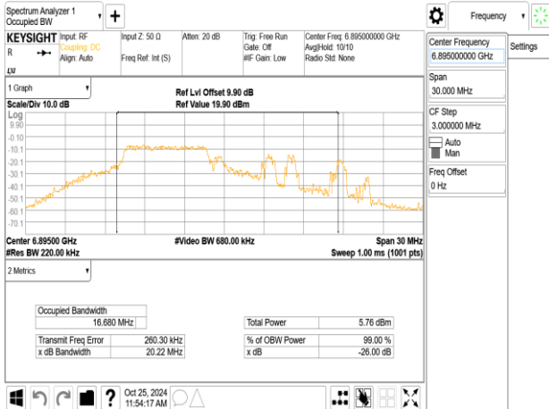
802.11be_20MHz_ChainA_6895MHz_RU106_53
