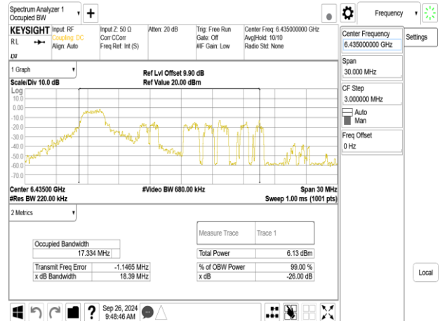
802.11be_20MHz_ChainB_6435MHz_RU52_37
