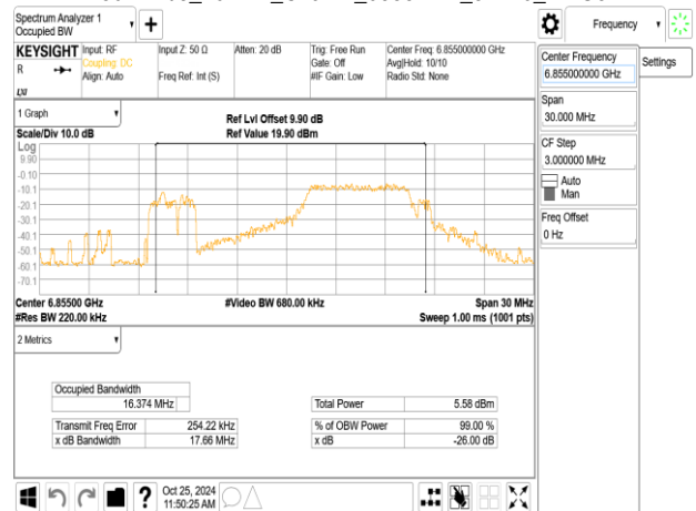
802.11be_20MHz_ChainB_6855MHz_RU106_54
