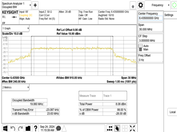
802.11be_20MHz_ChainB_6435MHz_106+26_MRU1
