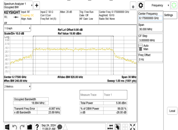
802.11be_20MHz_ChainB_6175MHz
