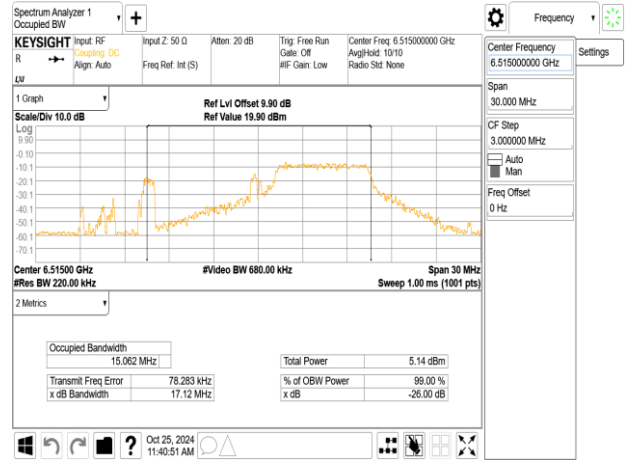
802.11be_20MHz_ChainB_6515MHz_RU106_54
