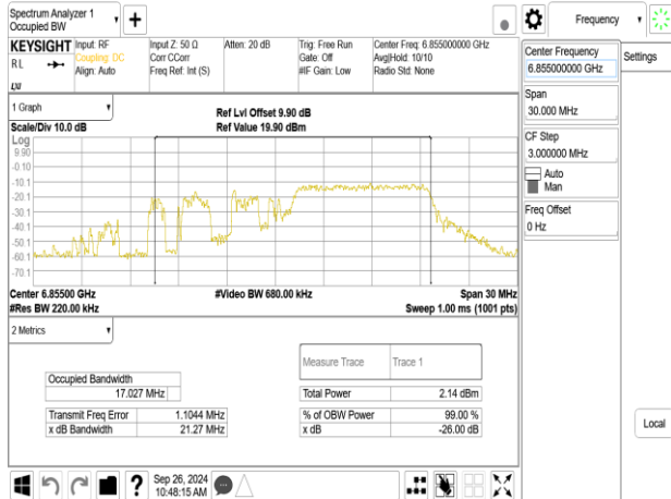
802.11be_20MHz_ChainA_6855MHz_RU26_8
