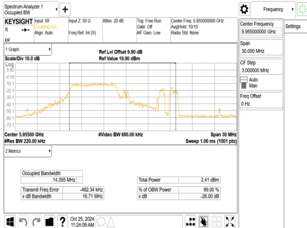
802.11be_20MHz_ChainB_5955MHz_RU106_53
