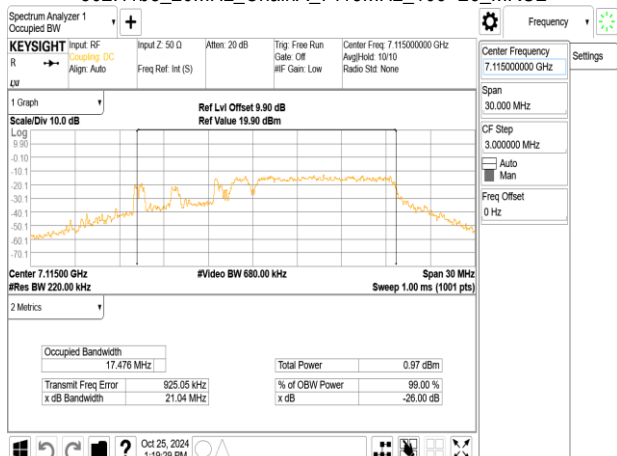
802.11be_20MHz_ChainA_7115MHz_52+26_MRU3
