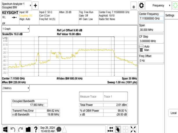
802.11be_20MHz_ChainB_7115MHz_RU26_8
