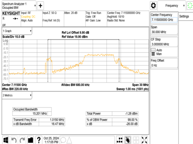
802.11be_20MHz_ChainB_7115MHz_RU106_54
