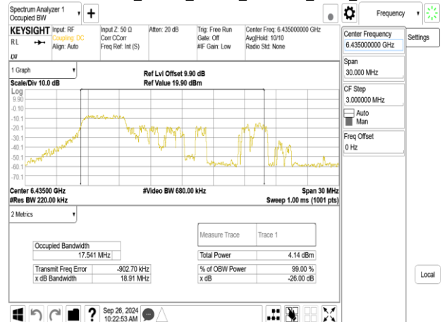
802.11be_20MHz_ChainB_6435MHz_RU52_37
