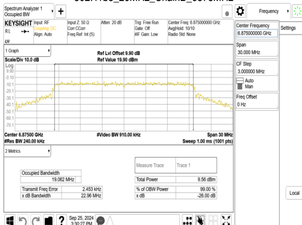
802.11be_20MHz_ChainB_6875MHz
