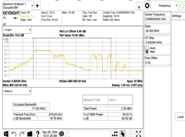
802.11be_20MHz_ChainB_6895MHz_RU52_37
