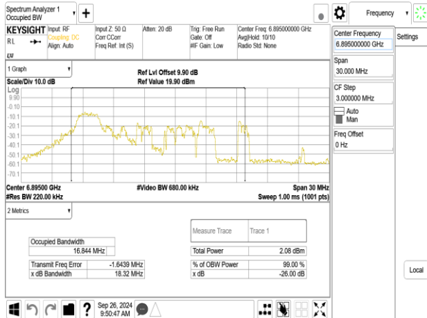
802.11be_20MHz_ChainB_6895MHz_RU52_37
