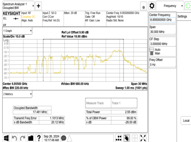
802.11be_20MHz_ChainA_6855MHz_RU52_40
