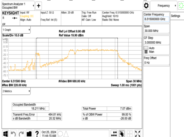
802.11be_20MHz_ChainB_6515MHz_106+26_MRJ2
