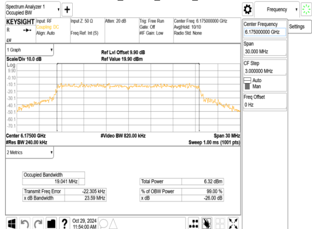
802.11ax_20MHz_ChainB_6175MHz
