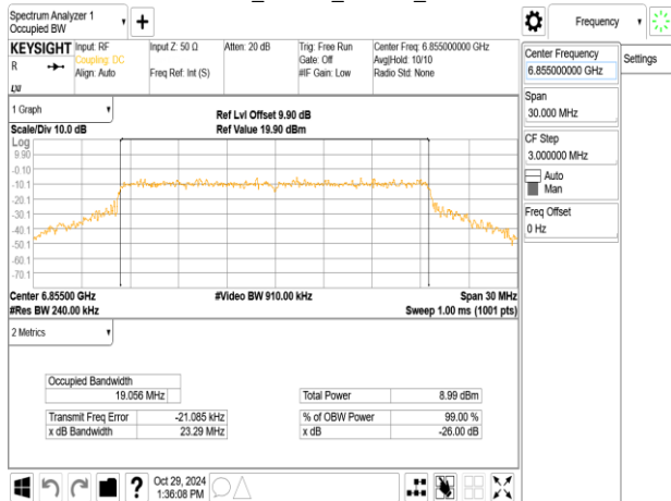
802.11ax_20MHz_ChainB_6855MHz_RU106_54
