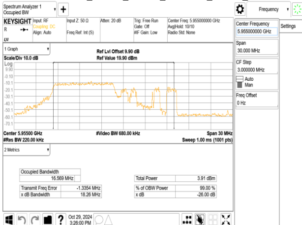
802.11ax_20MHz_ChainB_5955MHz_RU106_53
