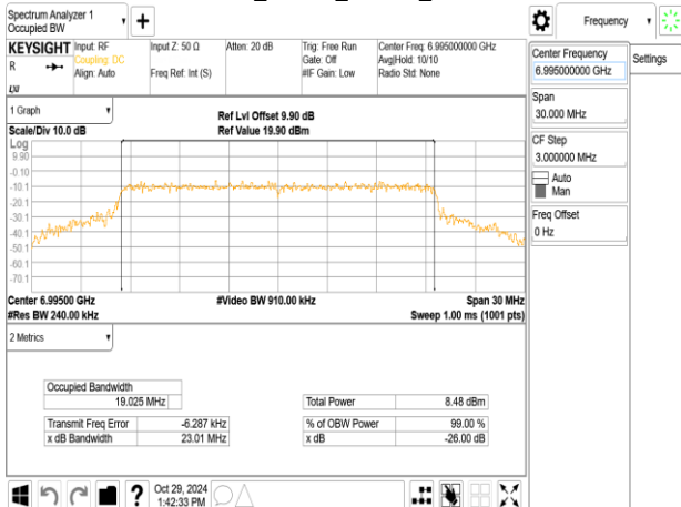
802.11ax_20MHz_ChainA_6995MHz
