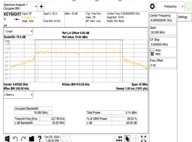
802.11ax_20MHz_ChainA_6855MHz
