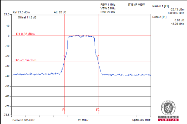
802.11ax (HE40)_Chain 1 / CH 187 (U-NII-8 Band)
