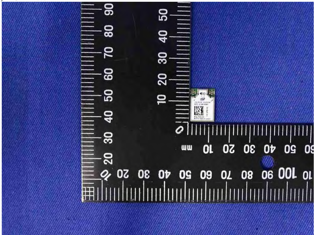
(40) EUT Photo
