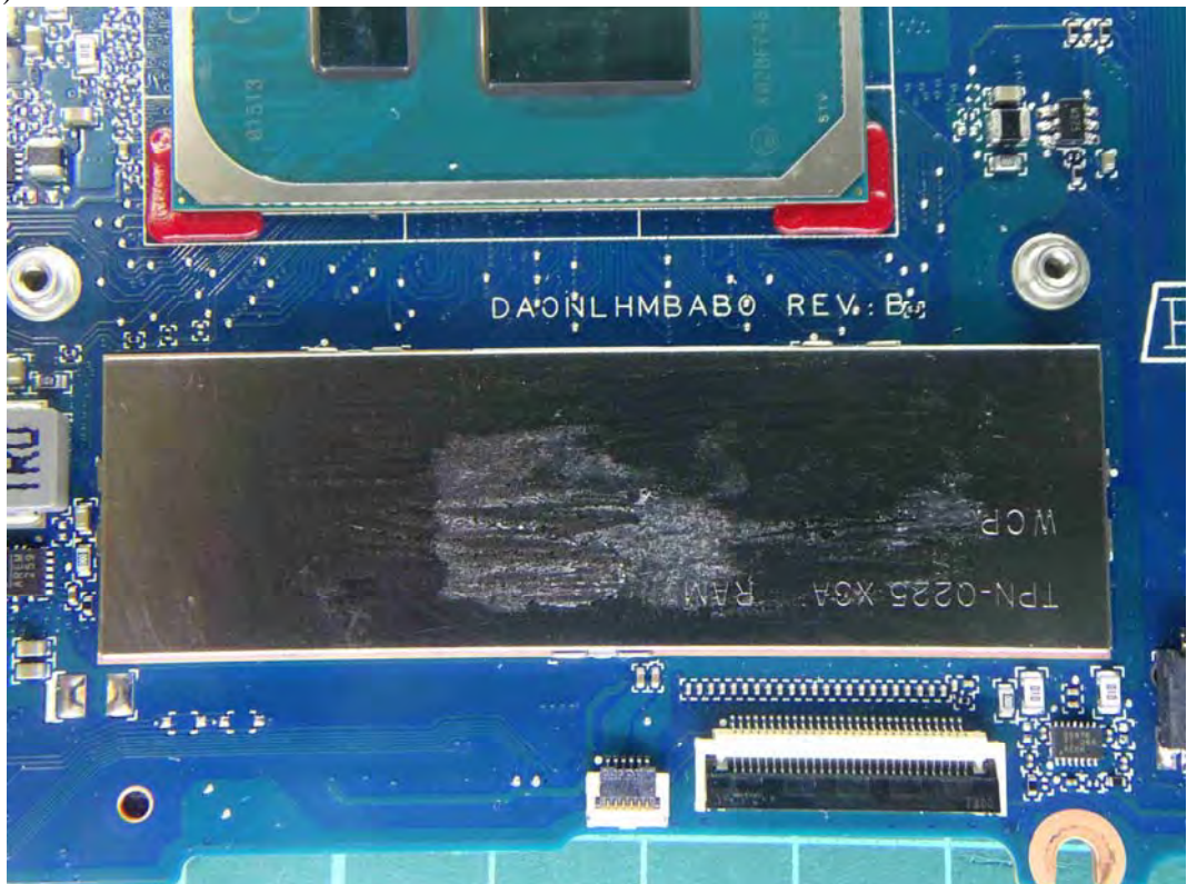
(58) EUT Photo
