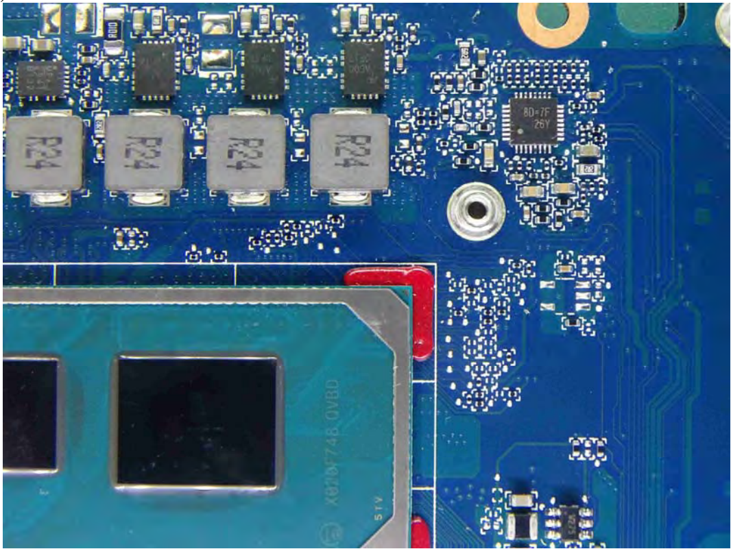
(56) EUT Photo
