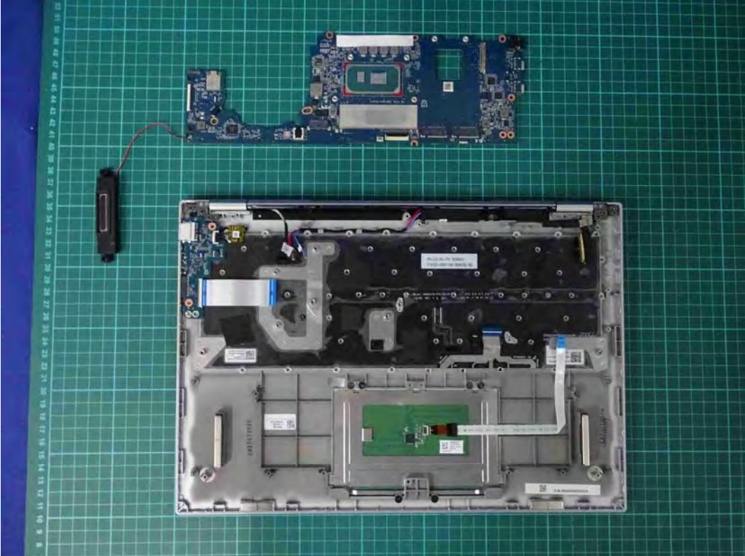
(49) EUT Photo
