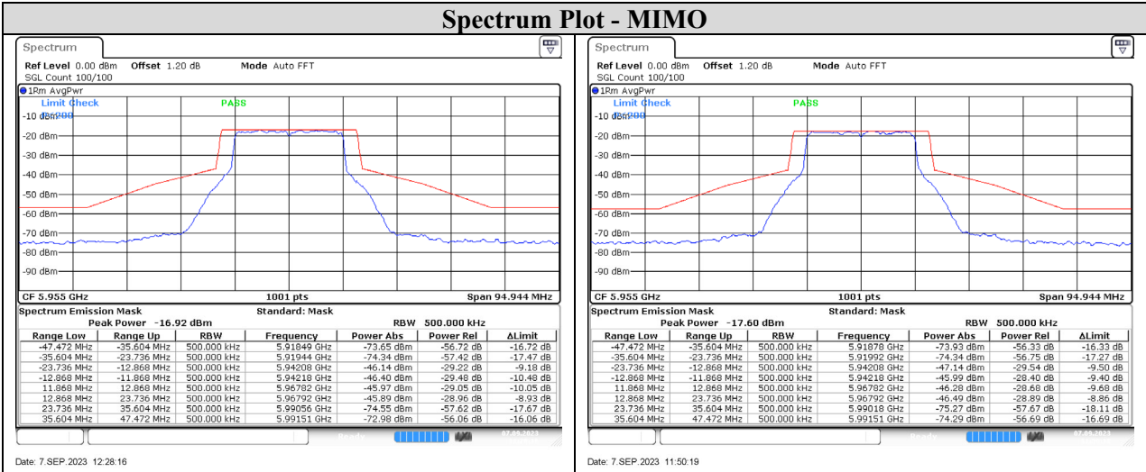
802.11ax (20 MHz) / 5955MHz / Chain A | 802.11ax (20 MHz) / 5955MHz / Chain B
