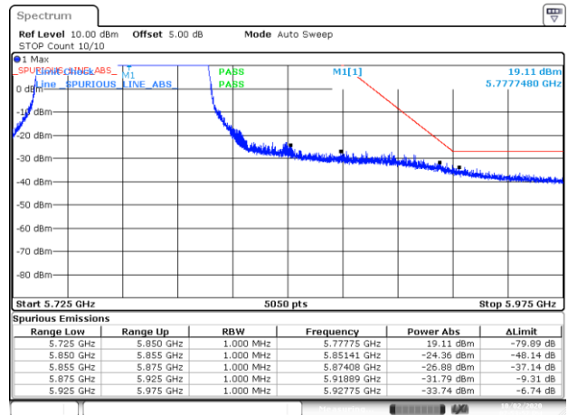
BE-NR-HIGH, SISO-A, 802.11ac80-HE0, Ch155
