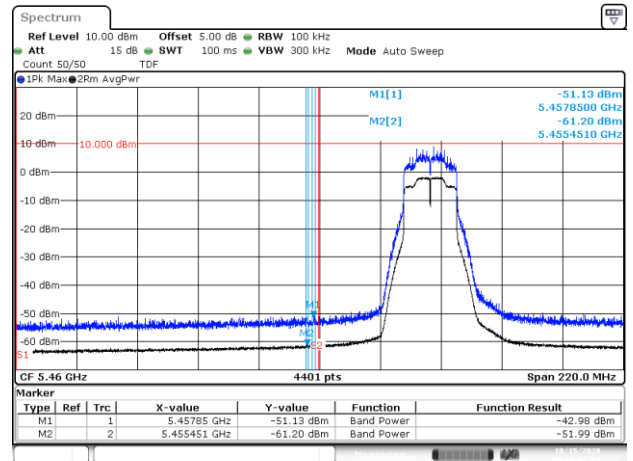
BE-R-LOW, MIMO-A, 802.11ax20-HE0, Ch100
