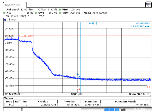
BE-NR-HIGH, MIMO-A, 802.11ax20-HE0, Ch140
