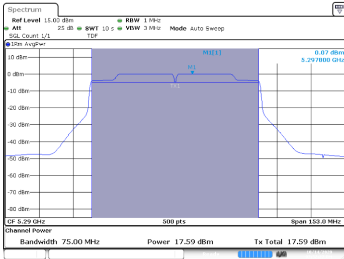
SISO A-802.11ac-80MHz-Ch58-5290MHz-VHT0
