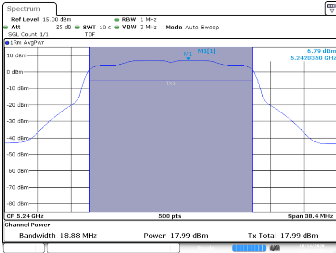
MIMO A-802.11ax-20MHz-Ch48-5240MHz-HE0
