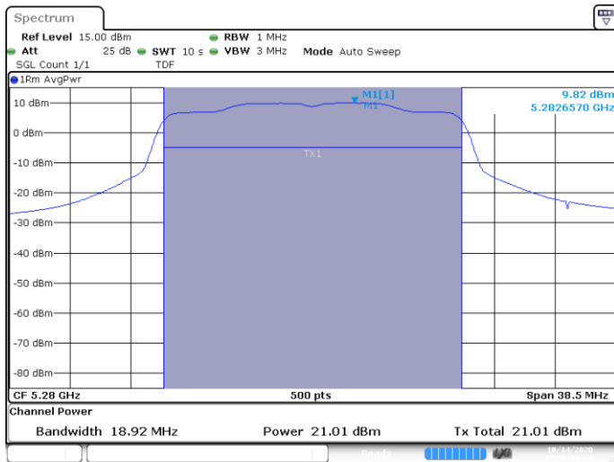
SISO A-802.11ax-20MHz-Ch56-5280MHz-HE0
