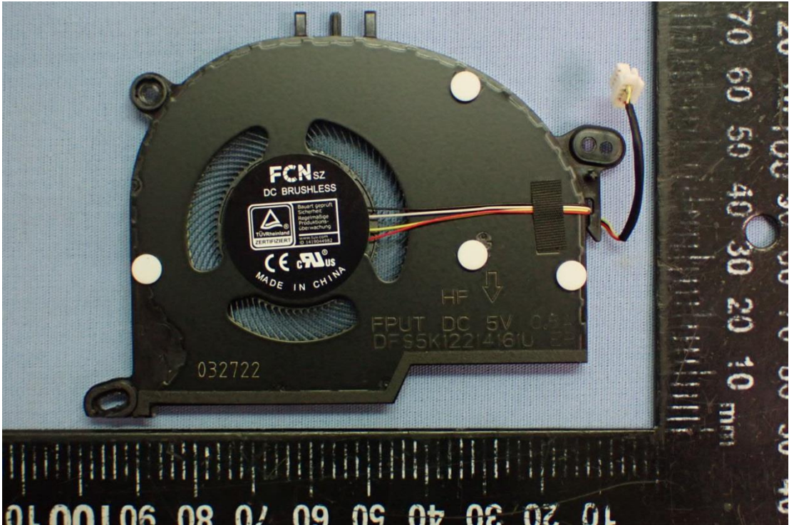
Figure 29 DC FAN
