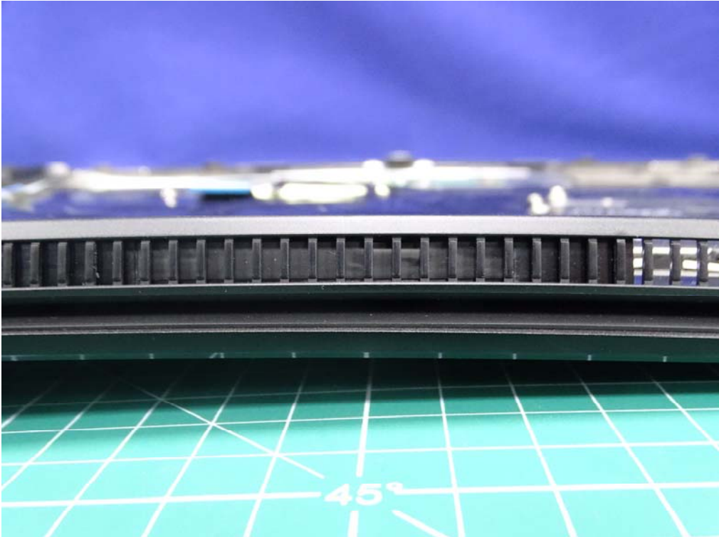
(67) EUT Photo
