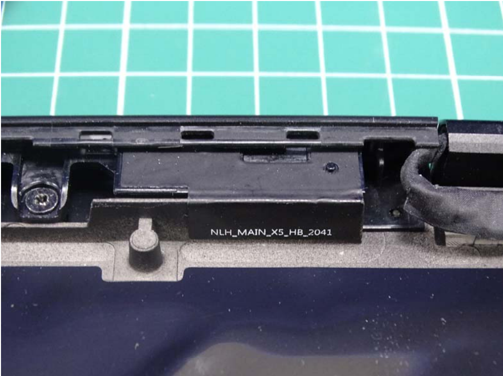
(64) EUT Photo
