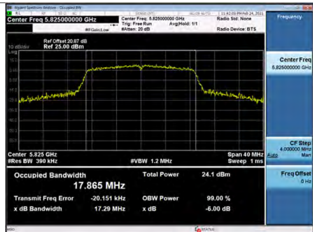
802.11n_HT20 UNII 3 (CH 165)
