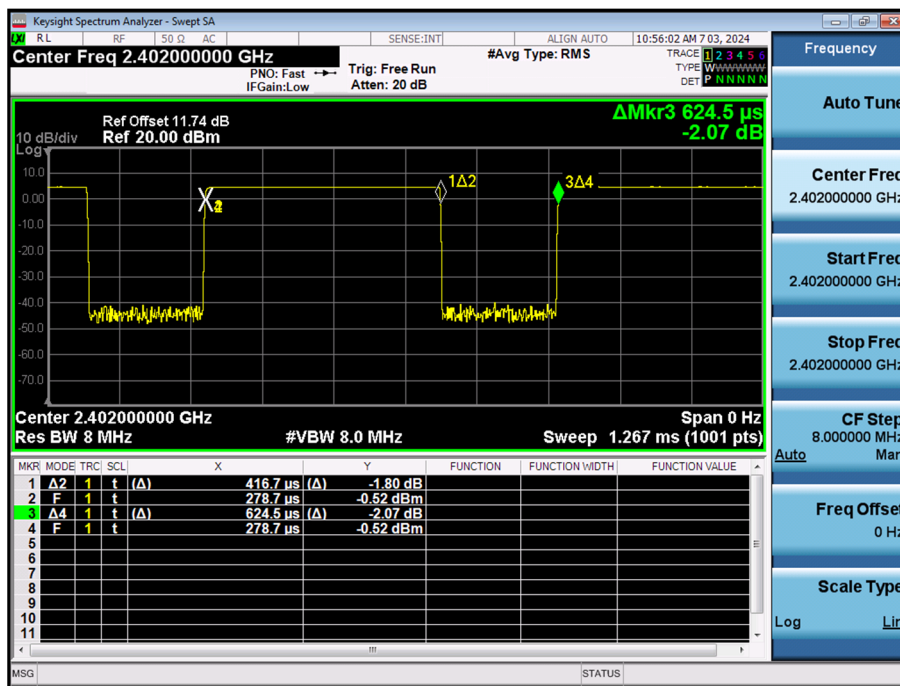
1 M Bit/s (37 Byte) Duty Cycle
