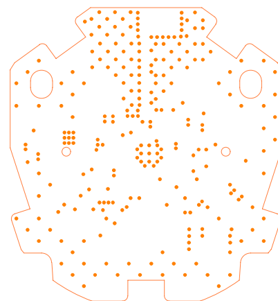
Bottom Via
