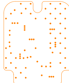
Bottom Via
