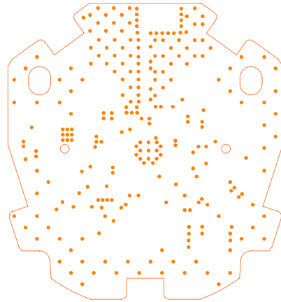
Top Via
