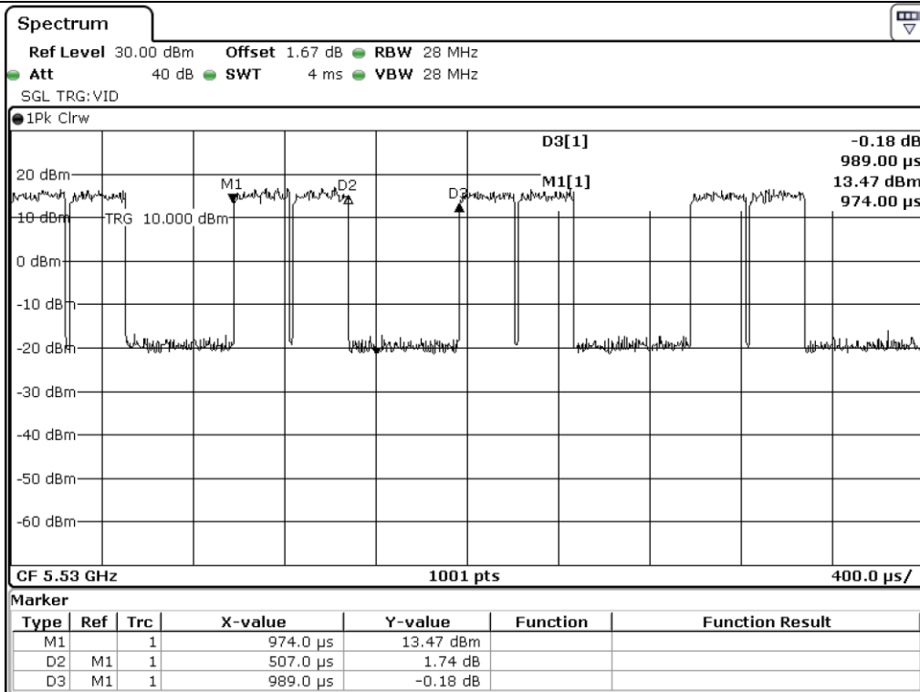
802.11 HT40
