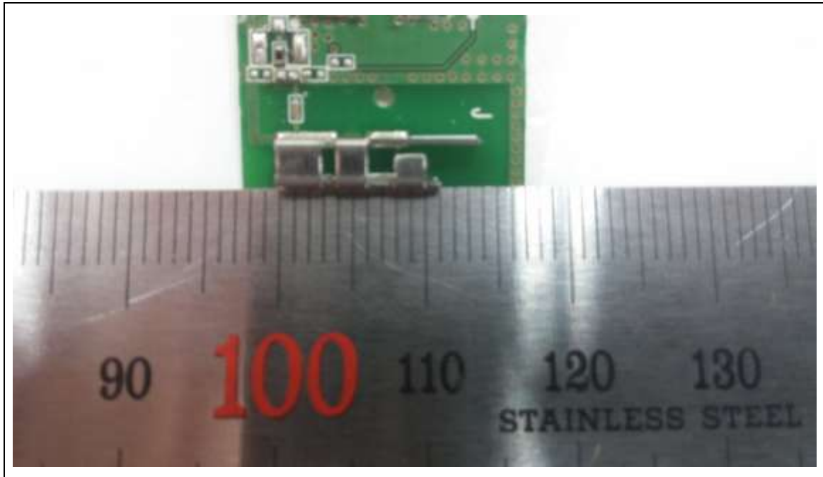
<TX/RX antenna>
