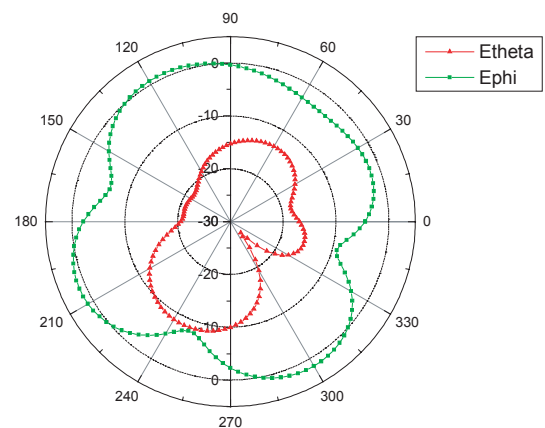
x - y cut (dBi)
