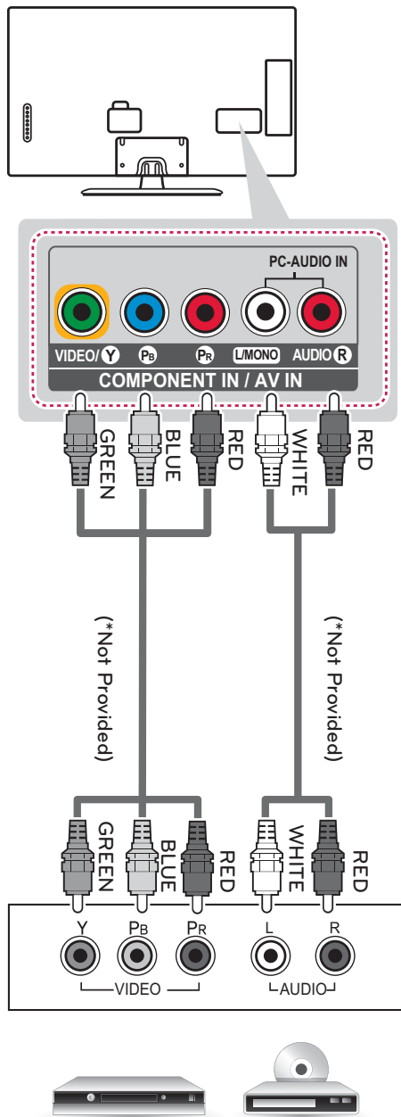
DVD / Blu-Ray / HD Cable Box
