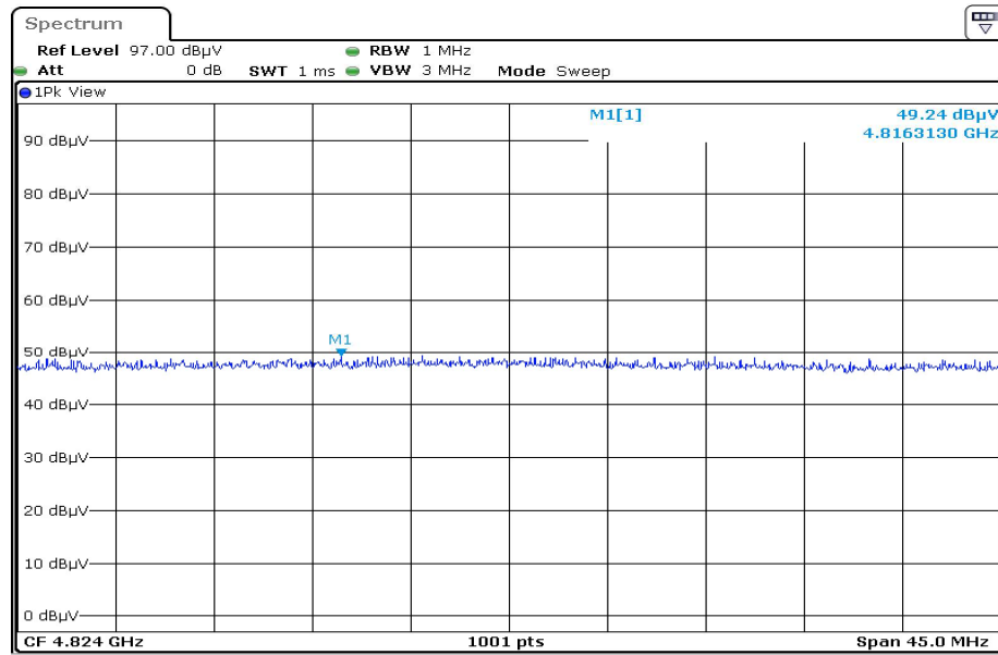
F1 X2 4824.0 Harmonic Vertical PEAK
