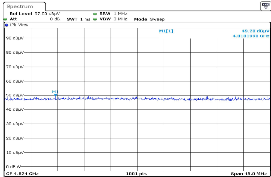
F1 X2 4824.0 Harmonic Vertical PEAK
