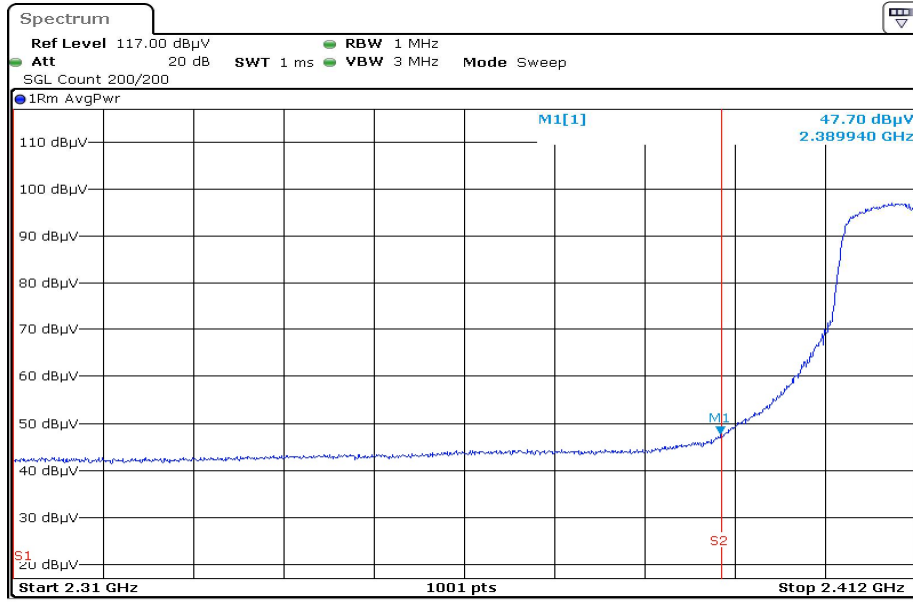
2412.0 F1 RestrictedBand Vertical AVG
