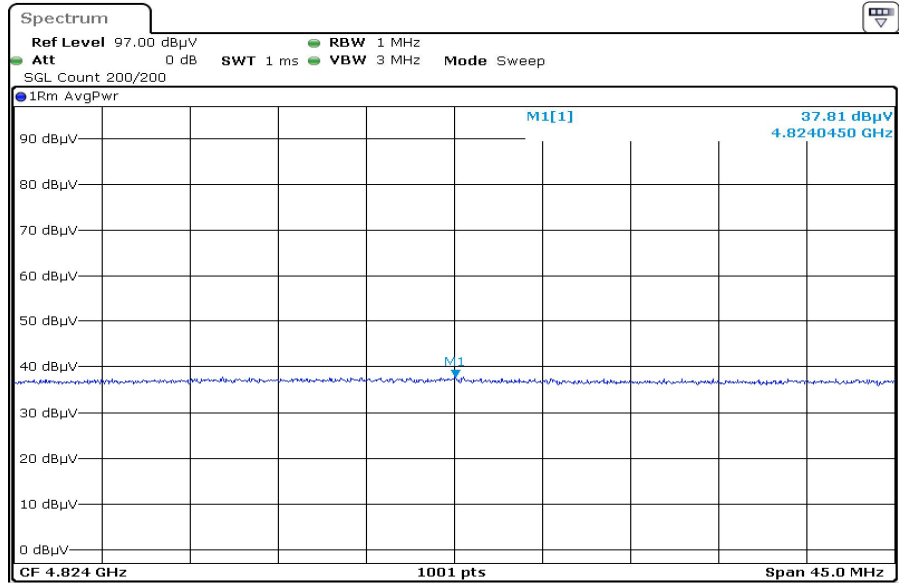
F1 X2 4824.0 Harmonic Vertical AVG
