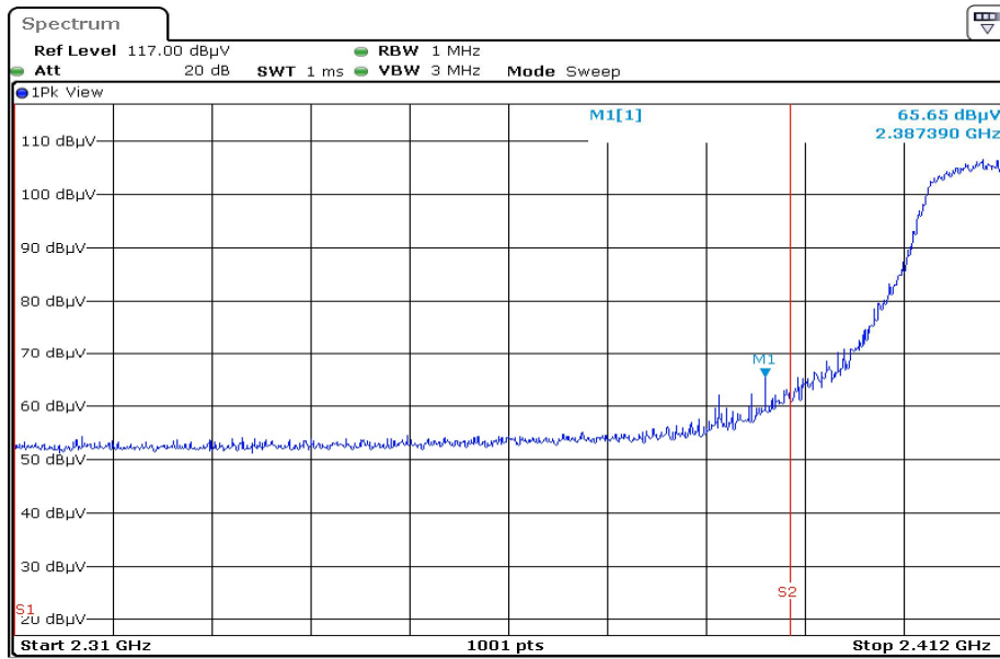
2412.0 F1 RestrictedBand Vertical PEAK
