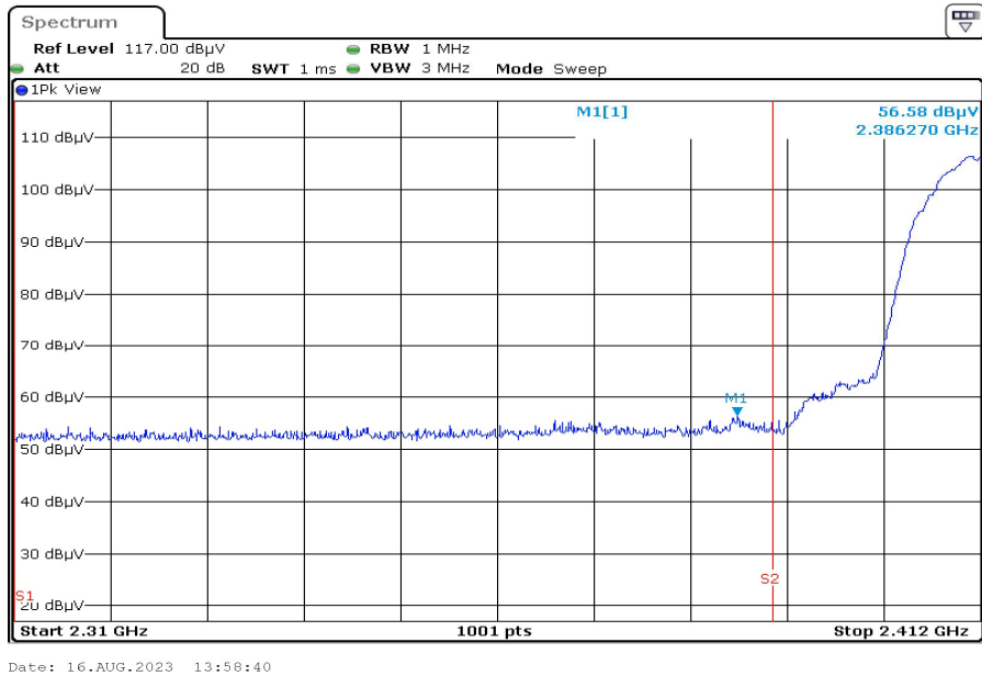
2412.0 F1 RestrictedBand Vertical PEAK
