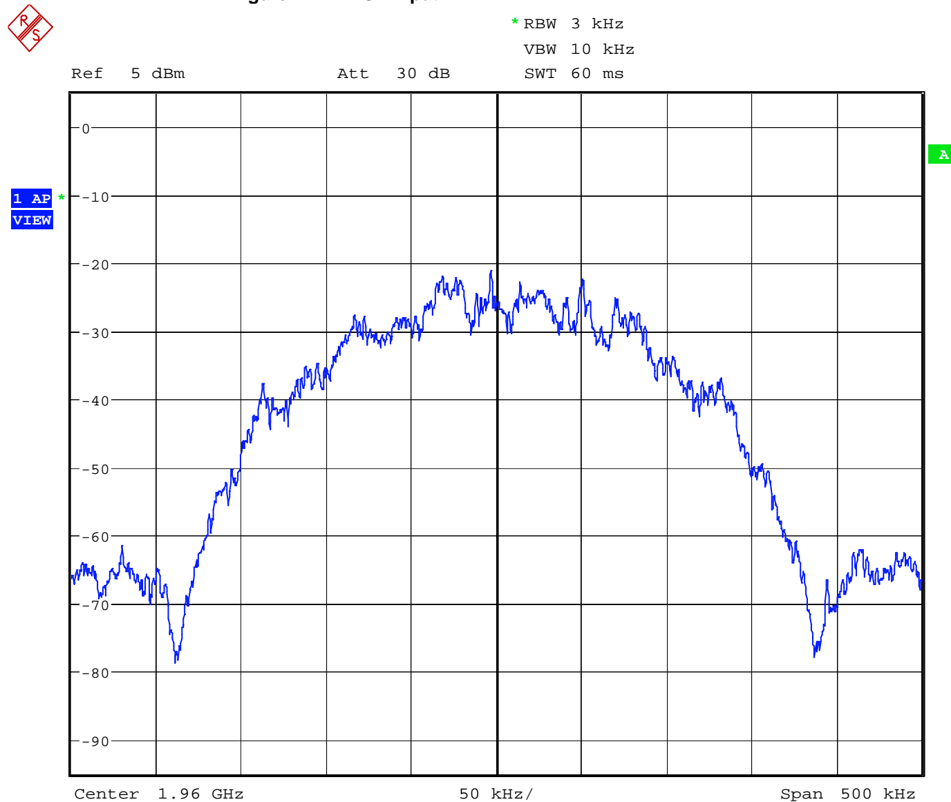
Figure 22 EDGE Input
