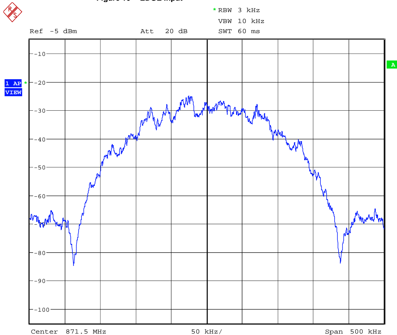
Figure 10 EDGE Input
