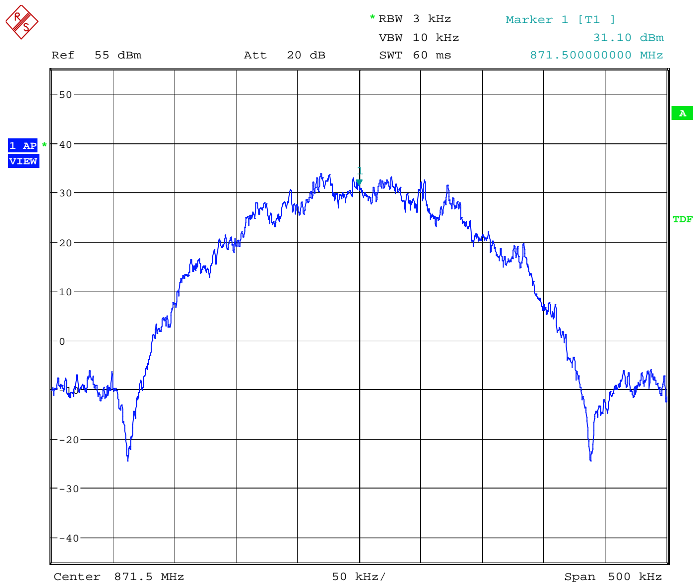
Figure 9 EDGE Output
