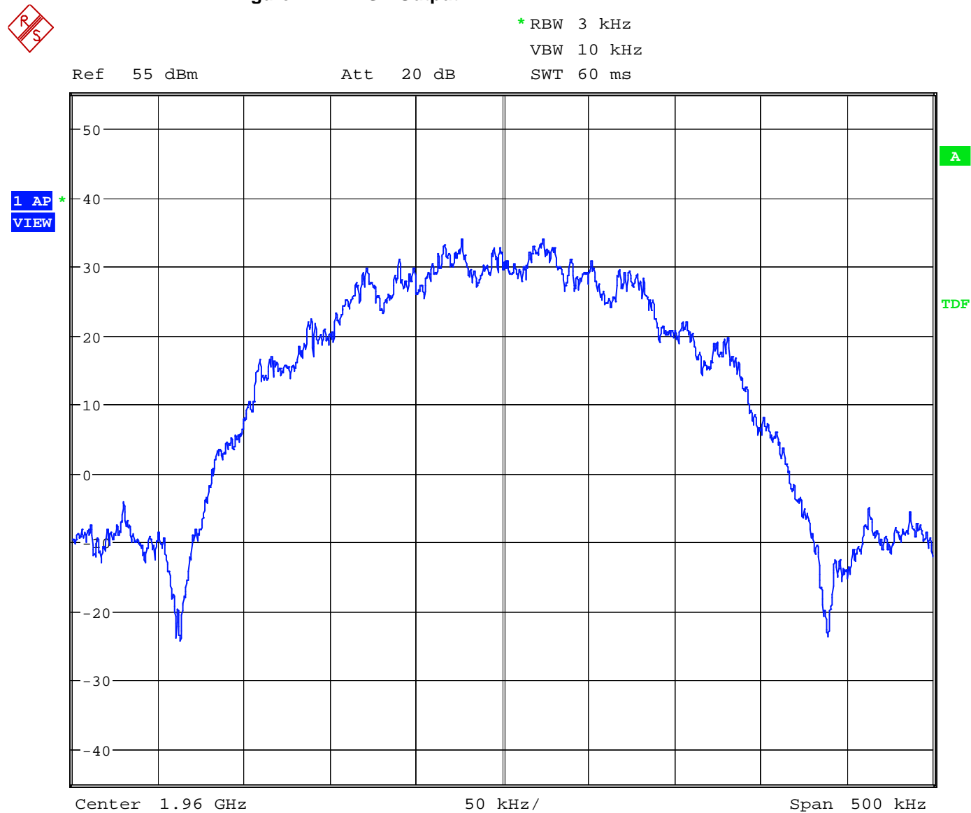
Figure 21 EDGE Output
