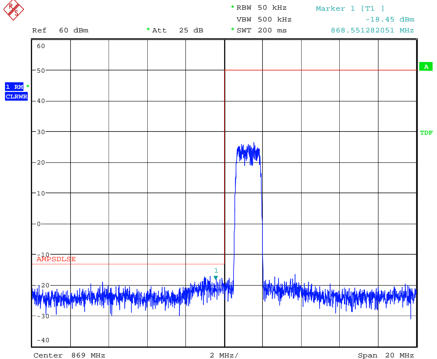
Figure 32 Edge
