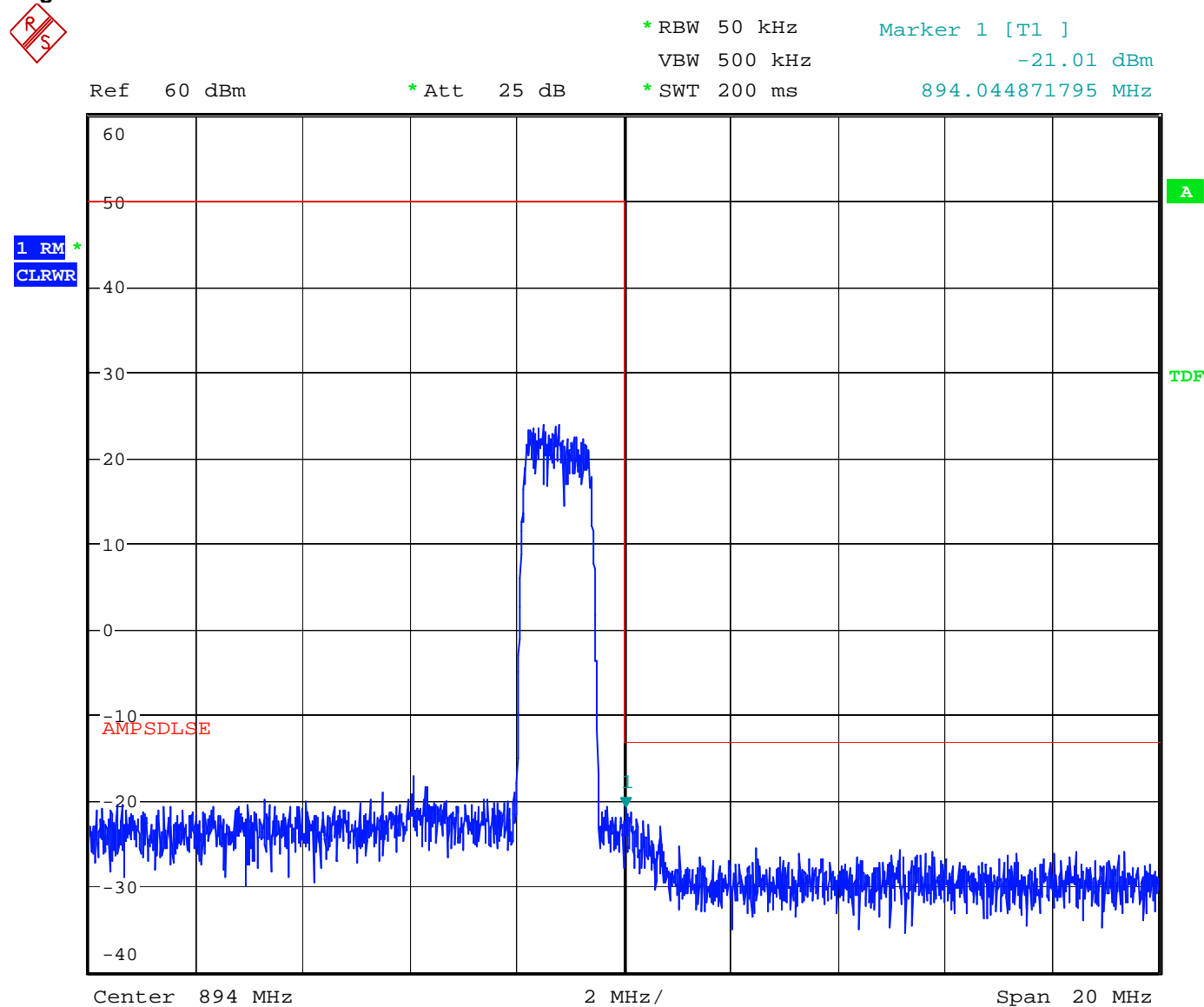
Figure 33 Edge
