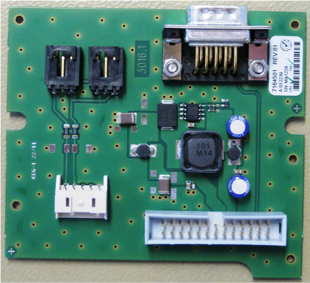
PCB P3016 7164501
