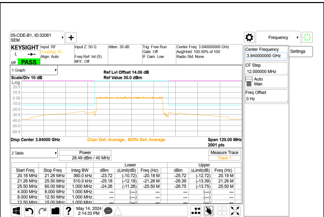
5G NR n77 40MHz BPSK Mid Channel RB105-0 Port A
