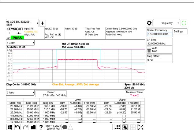
5G NR n77 40MHz BPSK Mid Channel RB105-0 Port B
