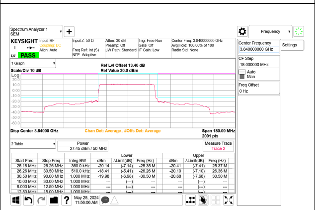
5G NR n77 50MHz BPSK Mid Channel RB128-0 Port B, ID: 32546
