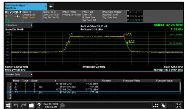
Figure 124 - 802.11ax HE40 SU VLP Maximum 26 dB EBW
