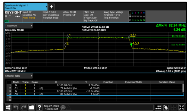
Figure 96 - 802.11ax HE80 SU SP Maximum 99% OBW
