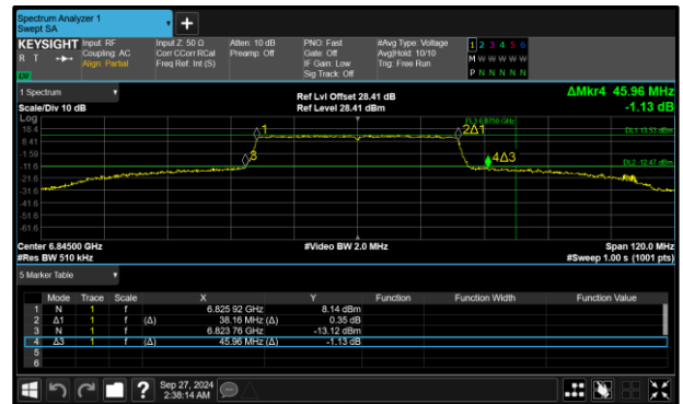
Figure 116 - 802.11ax HE40 SU SP Maximum 26 dB EBW
