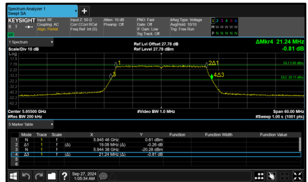
Figure 92 - 802.11ax HE20 SU SP Maximum 99% OBW
