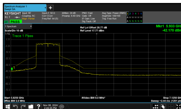
Figure 317 - A (Core 0) 802.11ax HE160 SU SP 6185 MHz (CH47)
