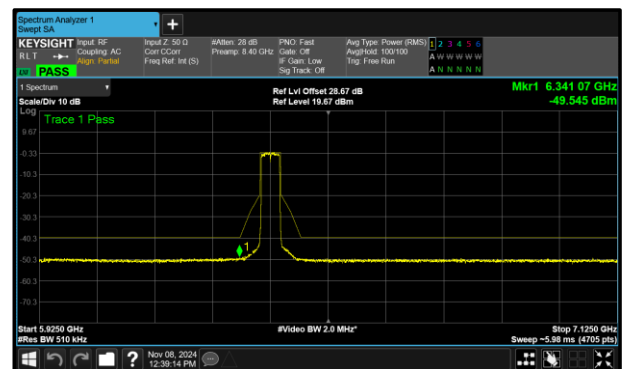
Figure 299 - B (Core 1) 802.11ax HE40 SU SP 6405 MHz (CH91)
