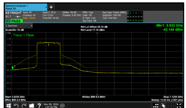
Figure 301 - B (Core 1) 802.11ax HE160 SU SP 6185 MHz (CH47)
