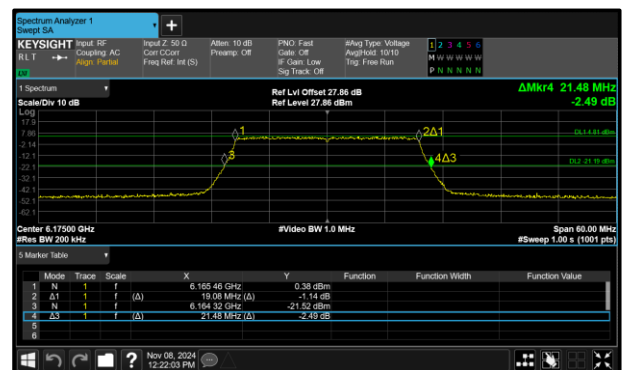
Figure 90 - 802.11ax HE20 SU SP Maximum 99% OBW
