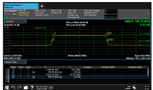
Figure 88 - 802.11ax HE160 SU LPI Maximum 99% OBW
