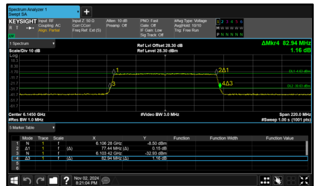
Figure 86 - 802.11ax HE80 SU LPI Maximum 99% OBW
