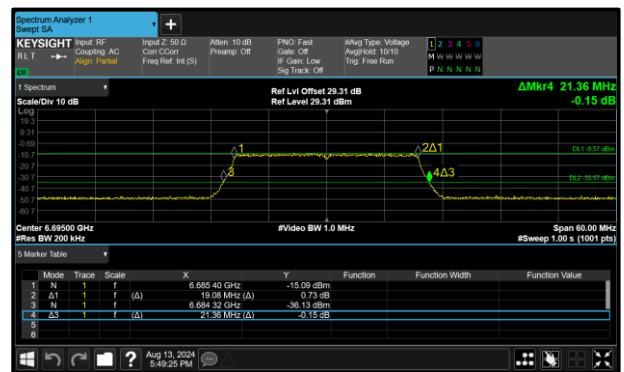
Figure 149 - 802.11ax HE20 SU VLP Maximum 99% OBW
