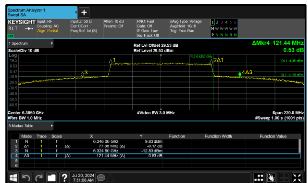
Figure 137 - 802.11ax HE80 SU SP Maximum 99% OBW
