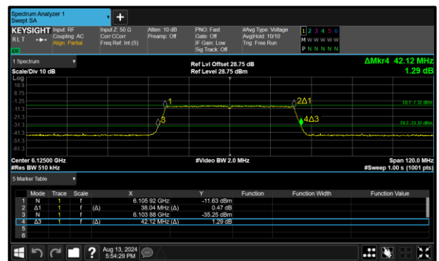
Figure 151 - 802.11ax HE40 SU VLP Maximum 99% OBW
