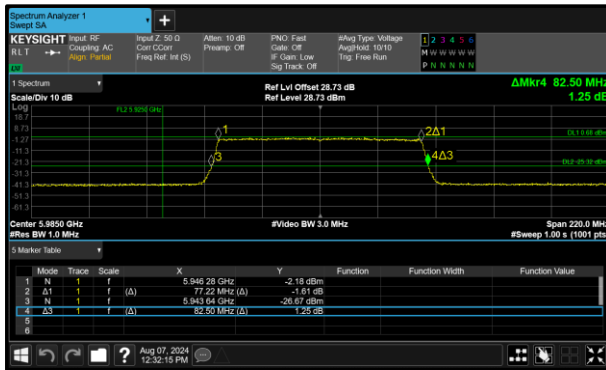
Figure 128 - 802.11ax HE80 SU LPI Minimum 99% OBW
