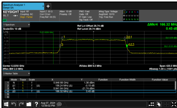
Figure 130 - 802.11ax HE160 SU LPI Minimum 99% OBW
