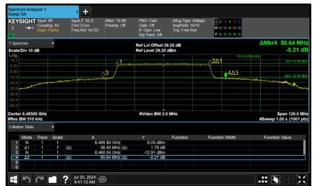
Figure 135 - 802.11ax HE40 SU SP Maximum 99% OBW
