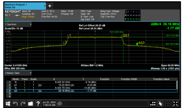
Figure 133 - 802.11ax HE20 SU SP Maximum 99% OBW
