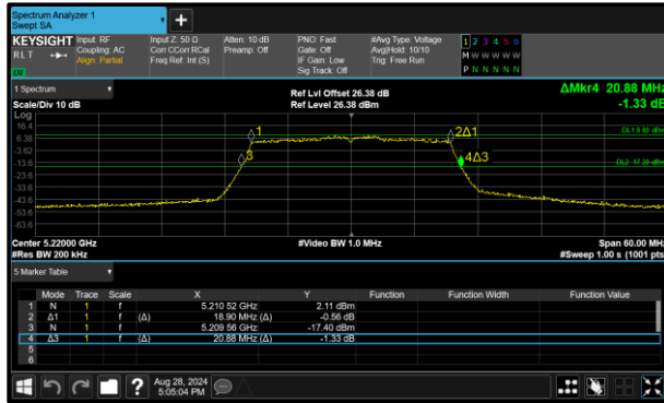
Figure 310 - 802.11ax HE20 SU Minimum 99% OBW
