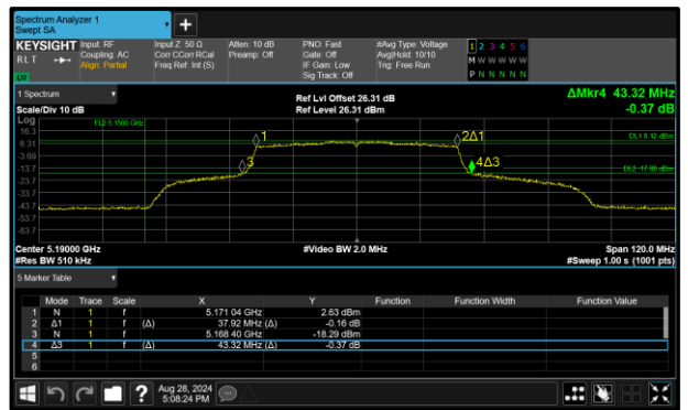
Figure 313 - 802.11ax HE40 SU Maximum 99% OBW
