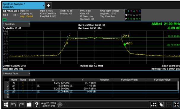
Figure 282 - 802.11ax HE20 SU Minimum 99% OBW
