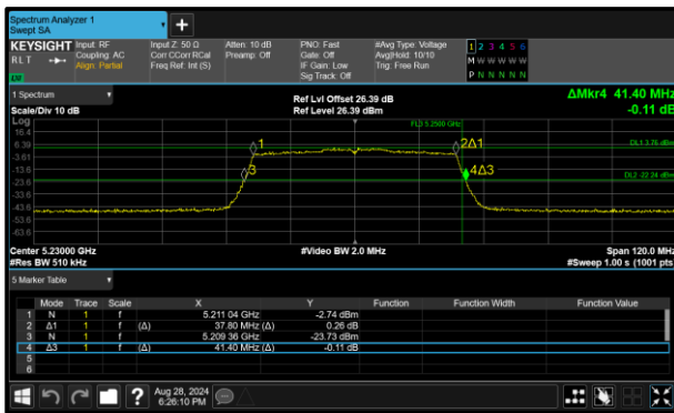
Figure 284 - 802.11ax HE40 SU Minimum 99% OBW
