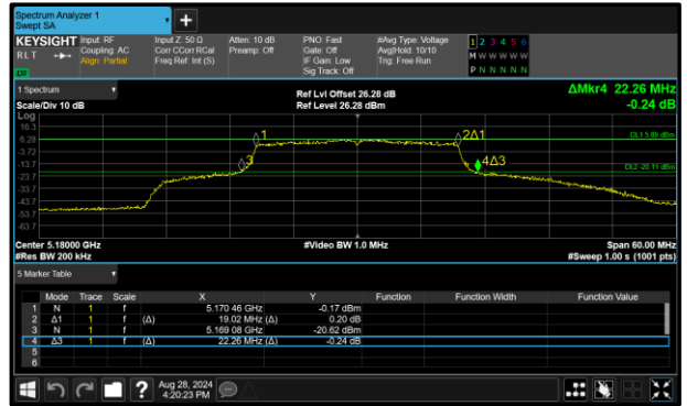
Figure 283 - 802.11ax HE20 SU Maximum 99% OBW
