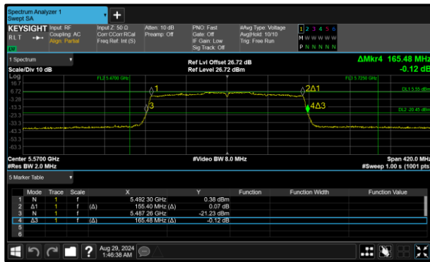
Figure 316 - 802.11ax HE160 SU Minimum 99% OBW
