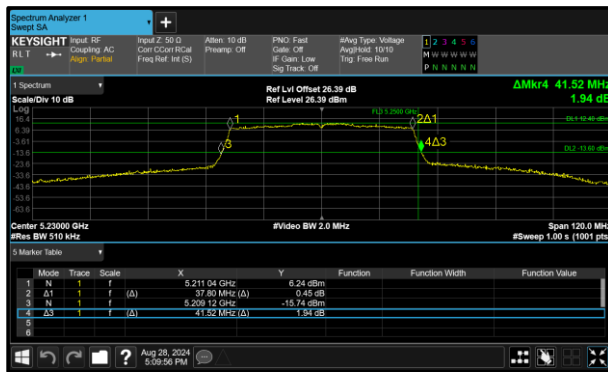
Figure 312 - 802.11ax HE40 SU Minimum 99% OBW
