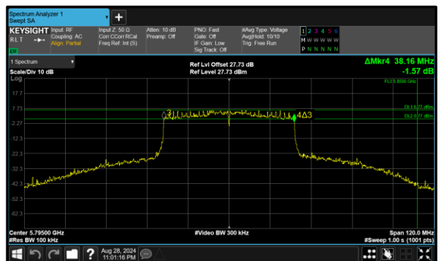
Figure 299 - 802.11ax HE40 SU Maximum 6 dB EBW
