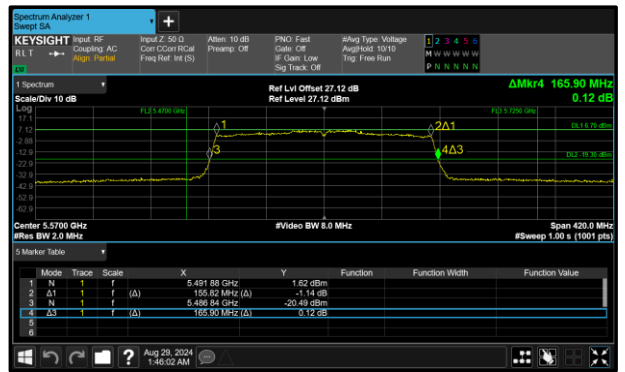
Figure 317 - 802.11ax HE160 SU Maximum 99% OBW
