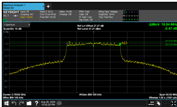
Figure 296 - 802.11ax HE20 SU Minimum 6 dB EBW
