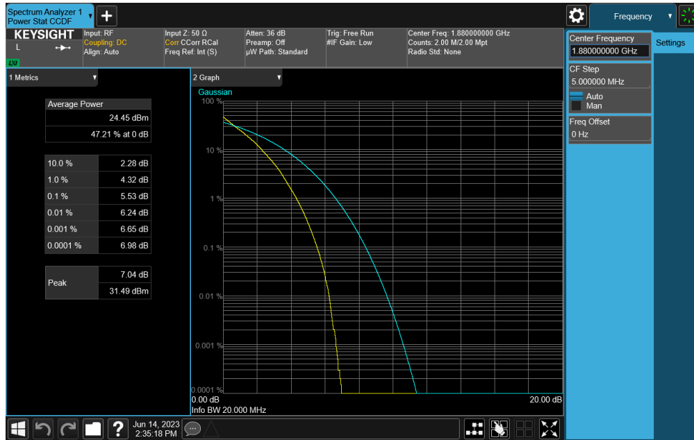
Plot 7-106. PAR Plot (LTE Band 2 - 20MHz QPSK - Full RB Configuration)
