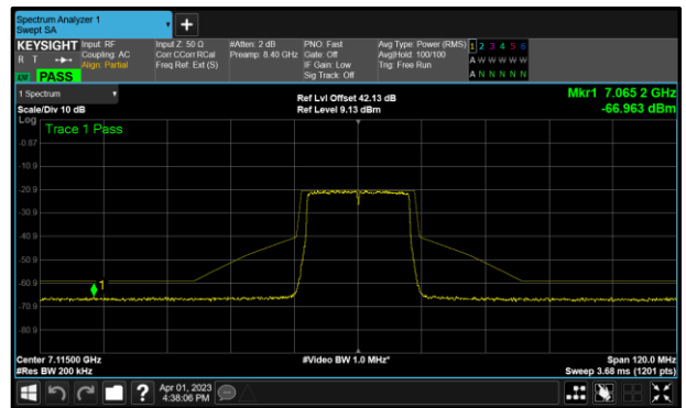
Figure 146 - A (Core 0) 802.11ax HE20 SU 7115 MHz (CH233)
