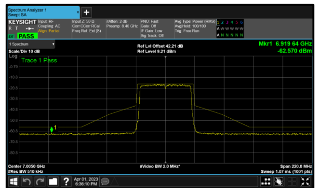
Figure 154 - A (Core 0) 802.11ax HE40 SU 7005 MHz (CH211)
