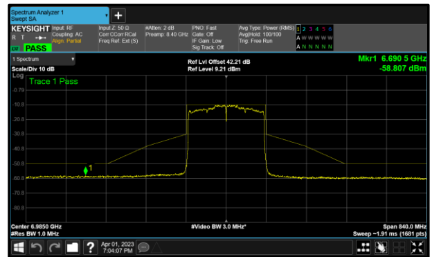
Figure 156 - A (Core 0) 802.11ax HE160 SU 6985 MHz (CH207)
