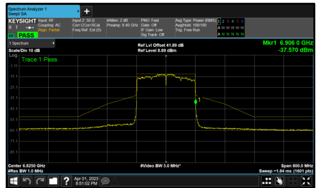
Figure 163 - A (Core 0) 802.11ax HE160 SU 6825 MHz (CH175)
