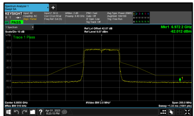
Figure 161 - A (Core 0) 802.11ax HE40 SU 6885 MHz (CH187)
