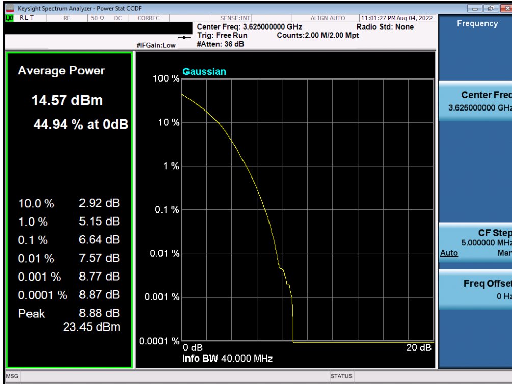
Plot 7-51. PAR Plot (NR Band n48 - 40MHz 256-QAM)
