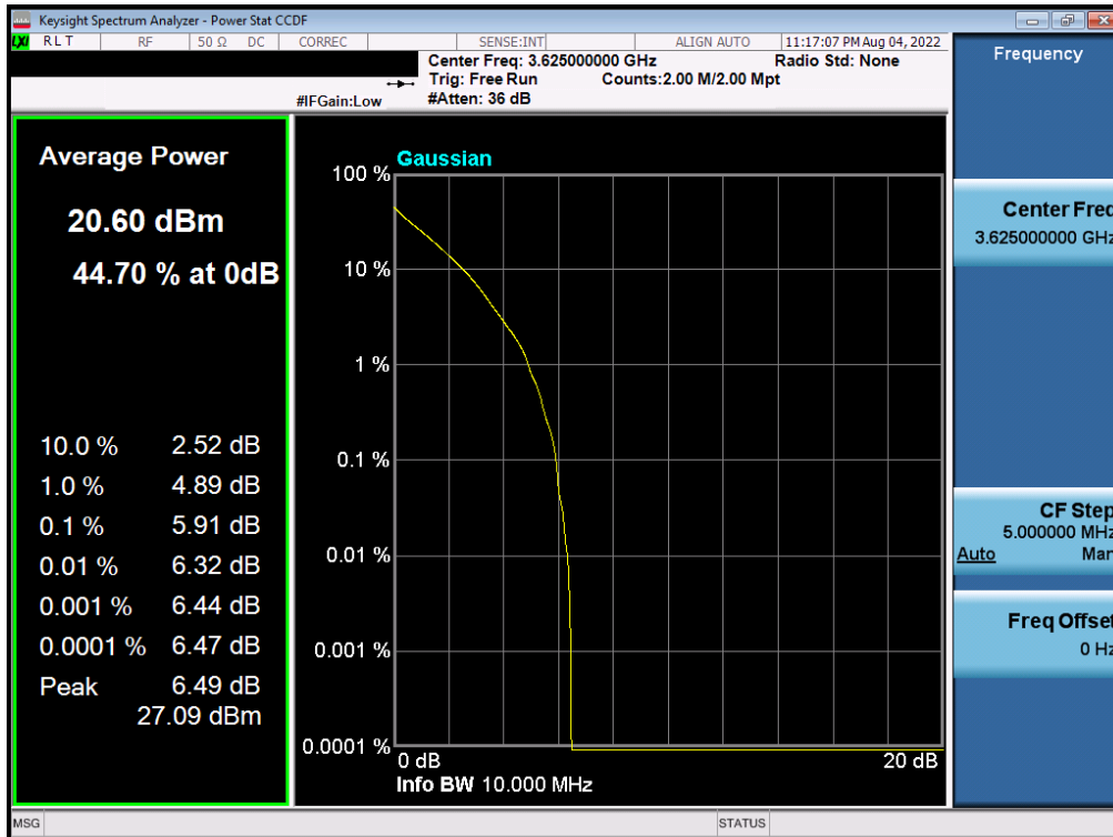
Plot 7-38. PAR Plot (NR Band n48 - 10MHz QPSK)
