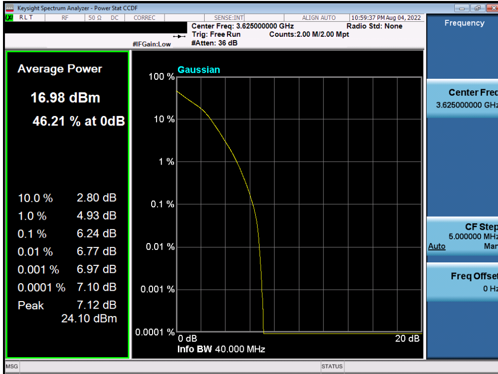
Plot 7-49. PAR Plot (NR Band n48 - 40MHz 16-QAM)
