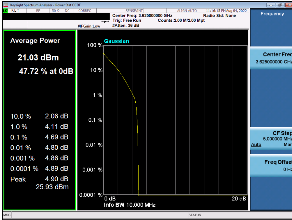
Plot 7-37. PAR Plot (NR Band n48 - 10MHz \pi/2 BPSK)
