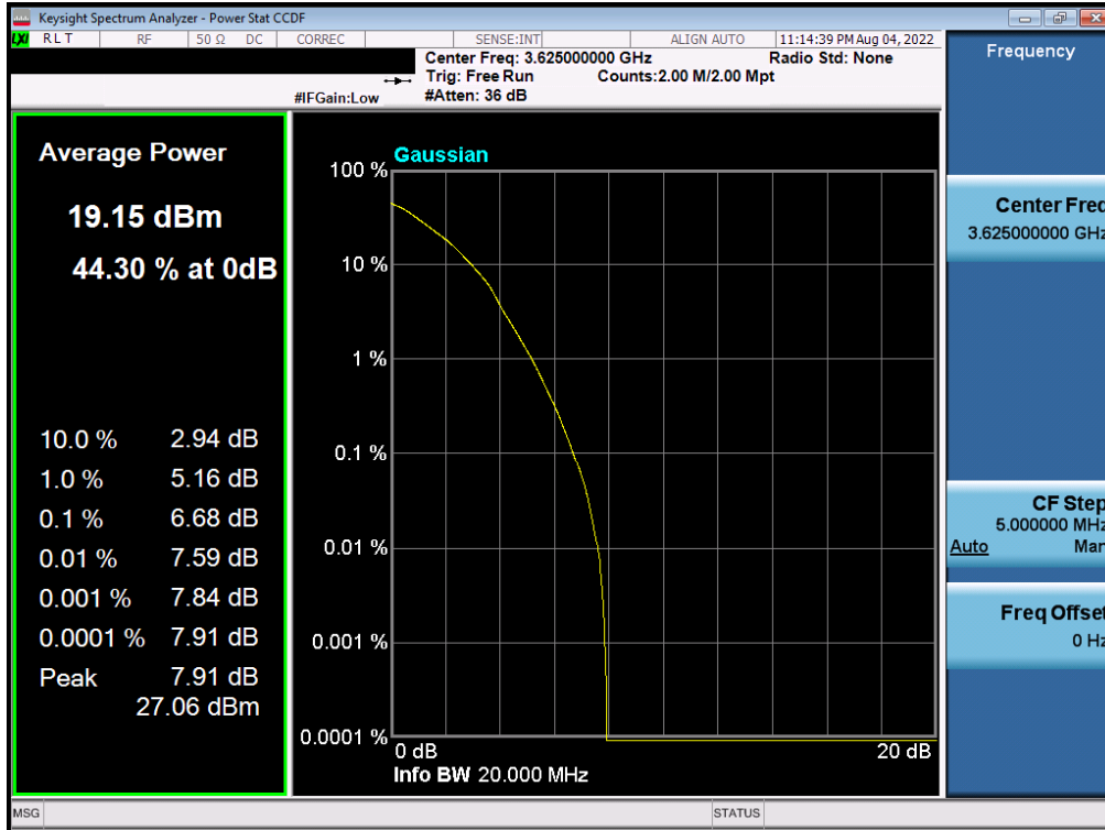
Plot 7-45. PAR Plot (NR Band n48 - 20MHz 64-QAM)
