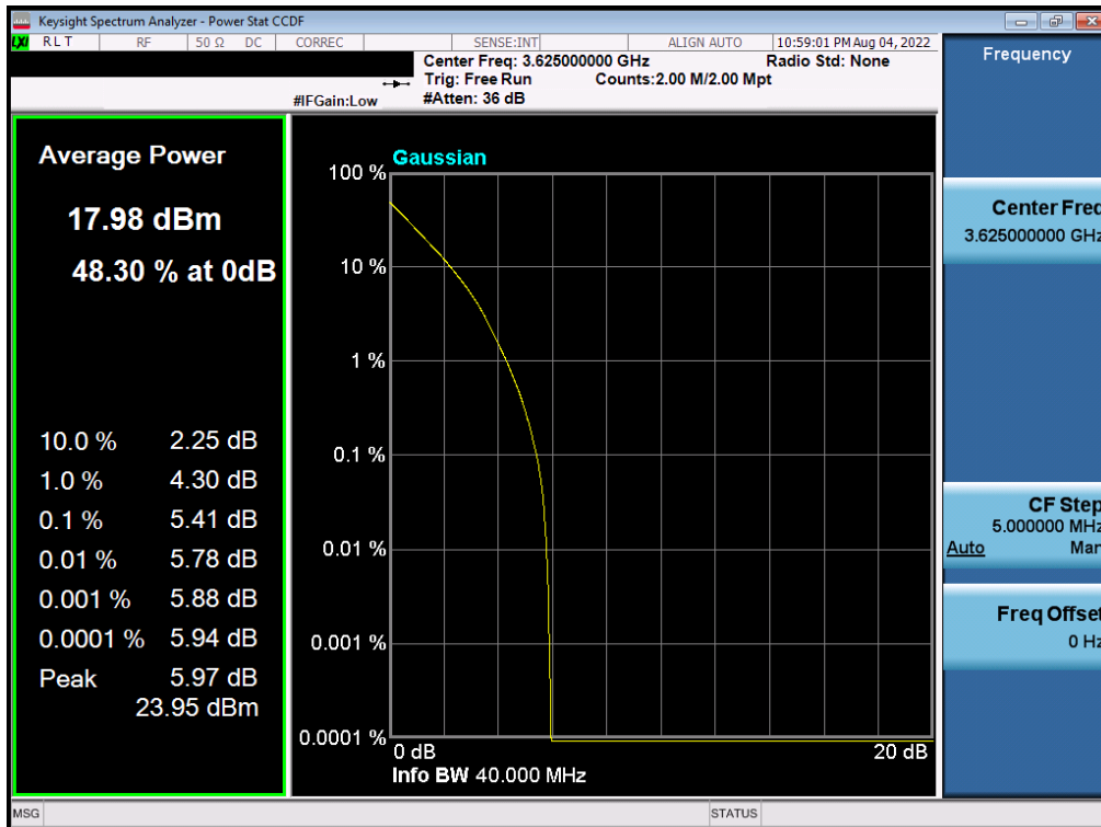
Plot 7-48. PAR Plot (NR Band n48 - 40MHz QPSK)
