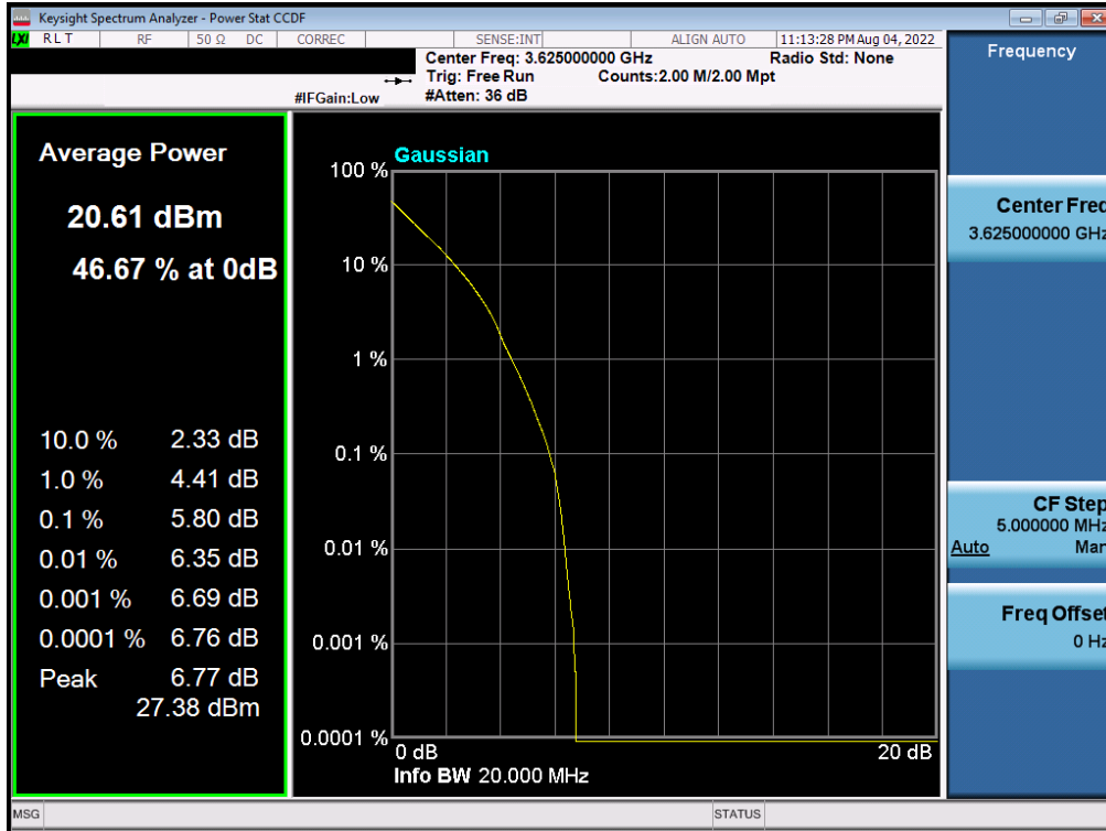
Plot 7-43. PAR Plot (NR Band n48 - 20MHz QPSK)
