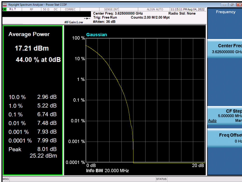
Plot 7-46. PAR Plot (NR Band n48 - 20MHz 256-QAM)
