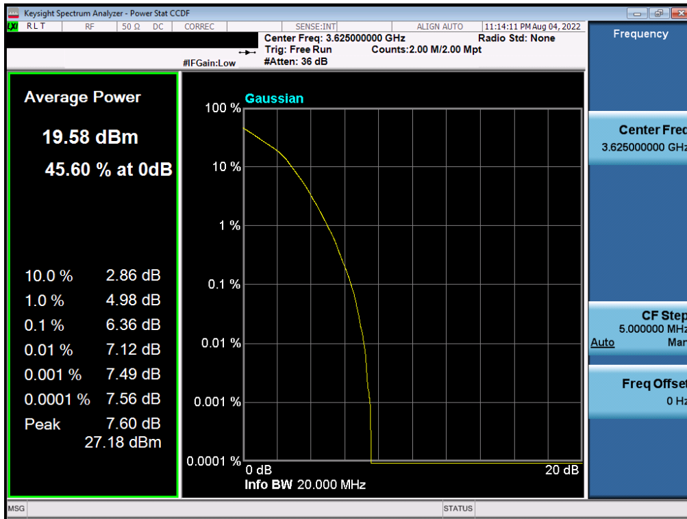
Plot 7-44. PAR Plot (NR Band n48 - 20MHz 16-QAM)
