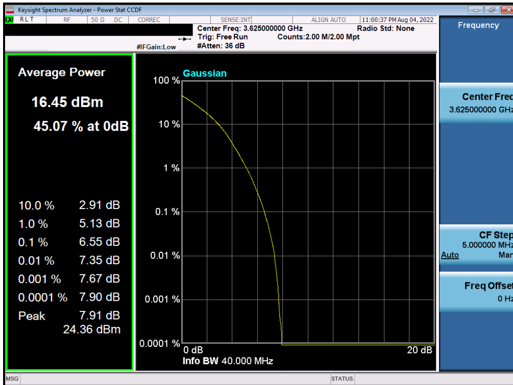
Plot 7-50. PAR Plot (NR Band n48 - 40MHz 64-QAM)
