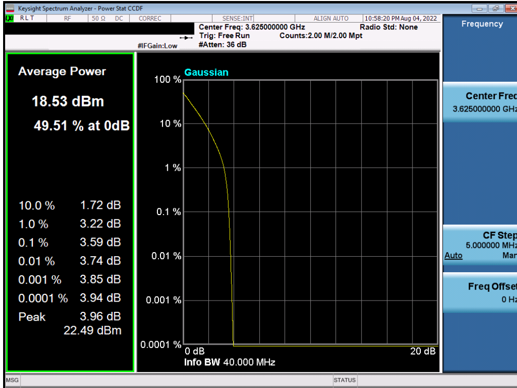
Plot 7-47. PAR Plot (NR Band n48 - 40MHz \pi/2 BPSK)
