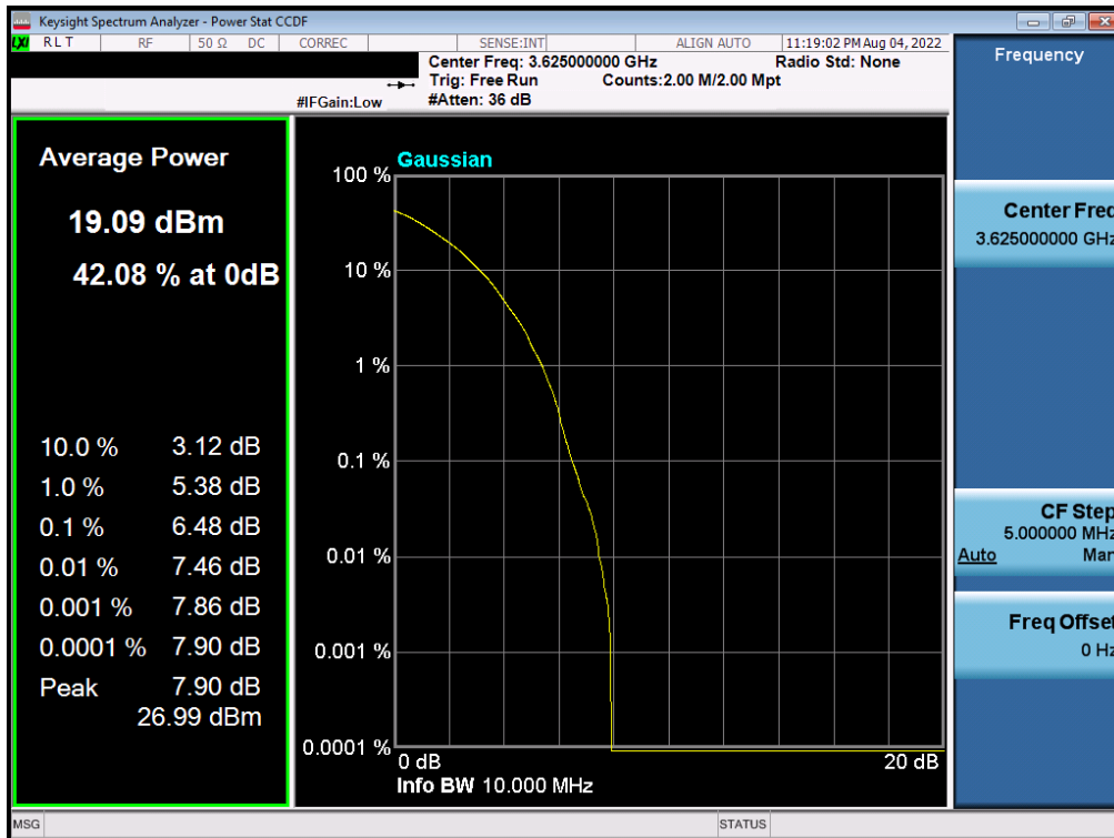
Plot 7-40. PAR Plot (NR Band n48 - 10MHz 64-QAM)
