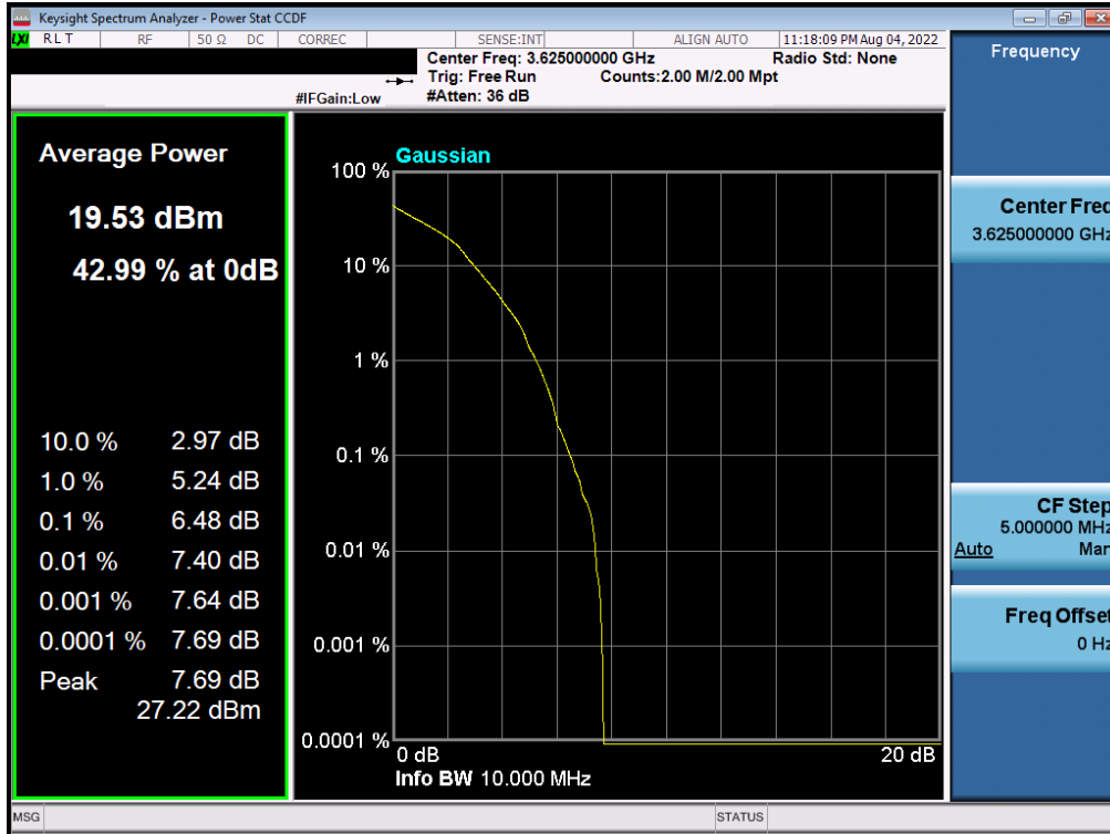
Plot 7-39. PAR Plot (NR Band n48 - 10MHz 16-QAM)
