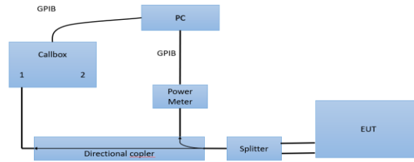
(d)Appendix E - Test Setup Photo 6
