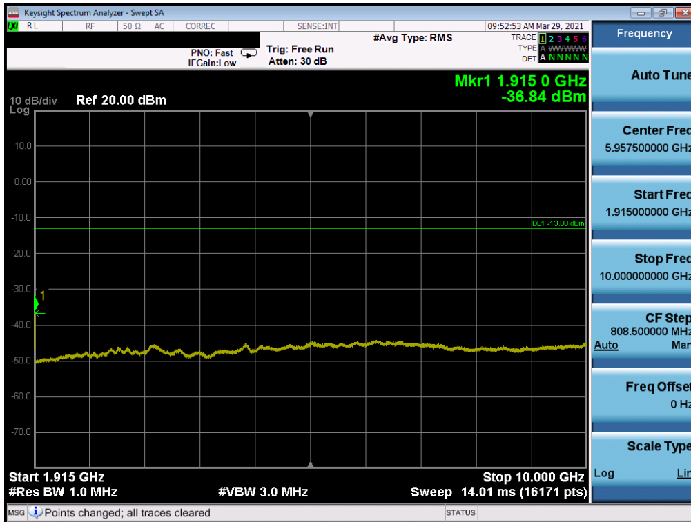
Plot 7-36. CSE (WCDMA Ch. 9538)
