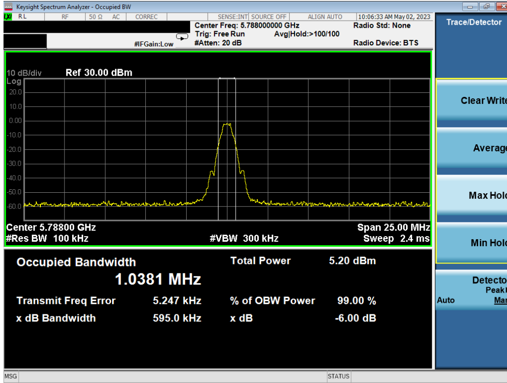
Plot 7-5. 6dB BW & 99% OBW (BDR, 5788MHz)
