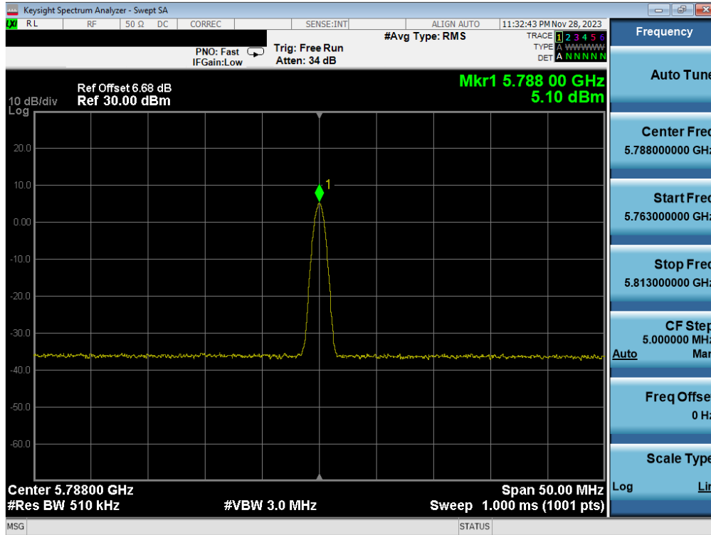
Plot 7-11. PSD (BDR, 5788MHz)
