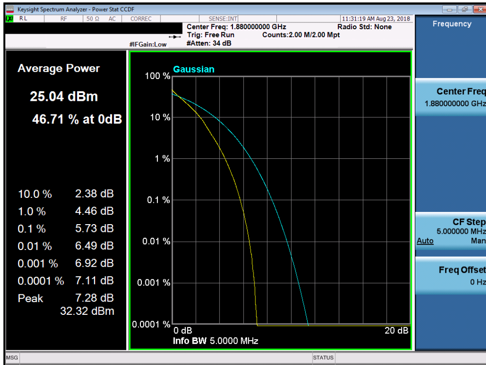
Plot 7-390. PAR Plot (Band 2 – 5.0MHz QPSK – RB Size 25)
