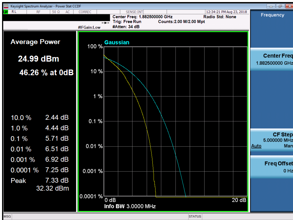
Plot 7-405. PAR Plot (Band 25 – 3.0MHz QPSK – RB Size 15)
