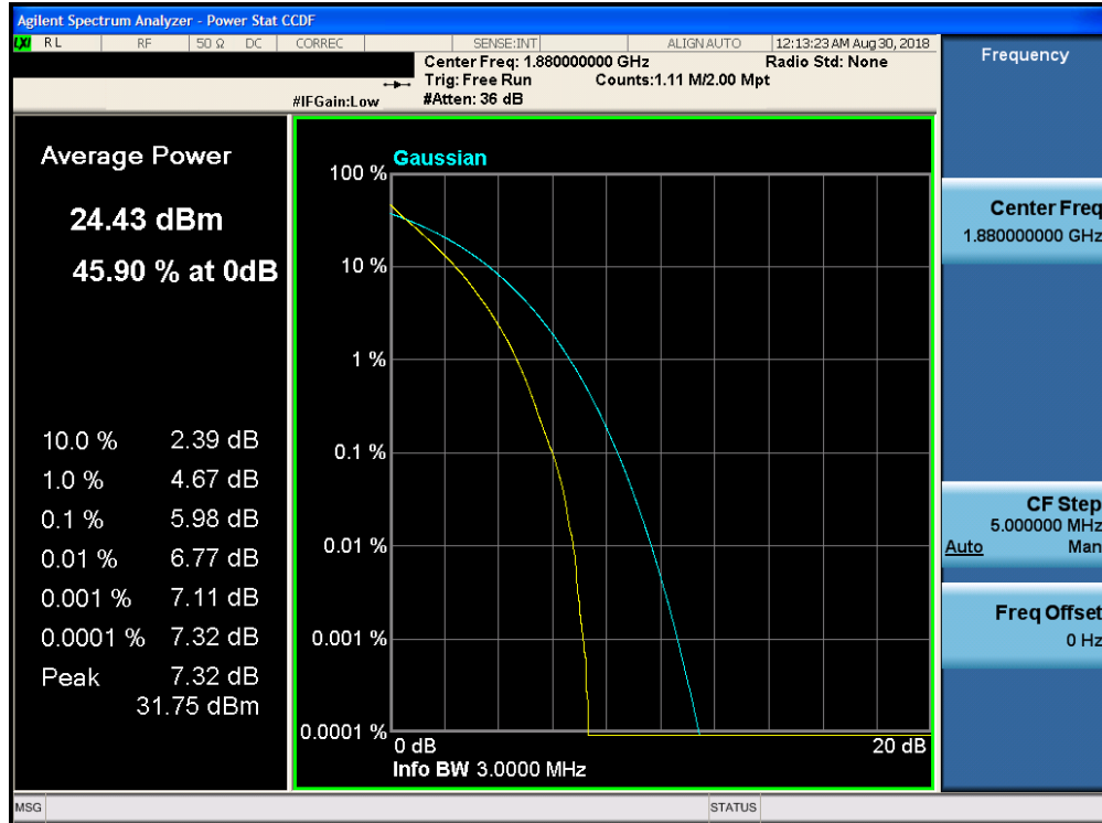
Plot 7-354. PAR Plot (Band 2 – 3.0MHz QPSK – RB Size 15)
