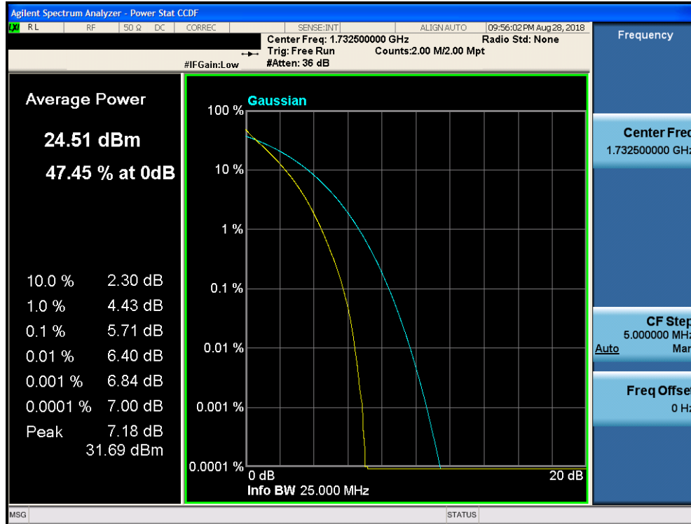
Plot 7-328. PAR Plot (Band 4 – 15.0MHz QPSK – RB Size 75)
