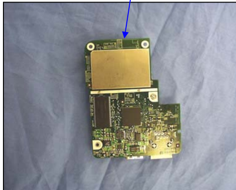
A1 antenna
