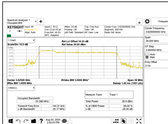
LTE B48 5MHz + 20MHz QPSK RB25-0 + RB100-0, ID:25780
