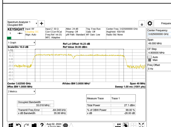
LTE B48 15MHz + 20MHz QPSK RB75-0 + RB100-0, ID:25780
