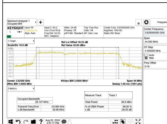
LTE B48 10MHz + 20MHz QPSK RB50-0 + RB100-0, ID:25780
