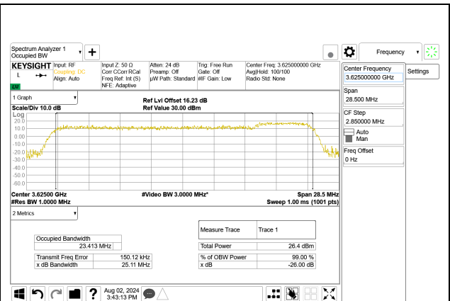
LTE B48 20MHz + 5MHz QPSK RB100-0 + RB25-0, ID:25780
