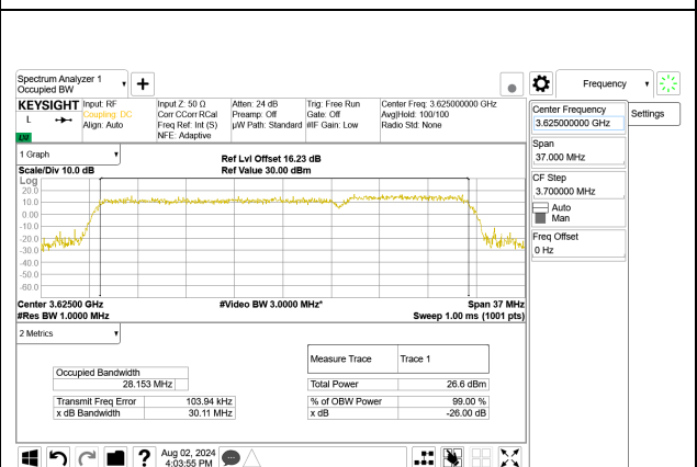
LTE B48 20MHz + 10MHz QPSK RB100-0 + RB50-0, ID:25780
