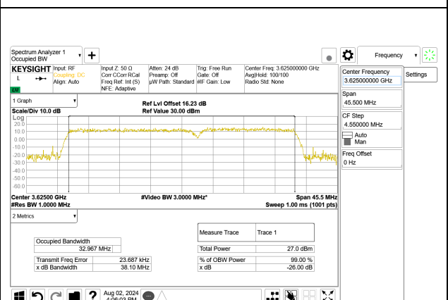
LTE B48 20MHz + 15MHz QPSK RB100-0 + RB75-0, ID:25780
