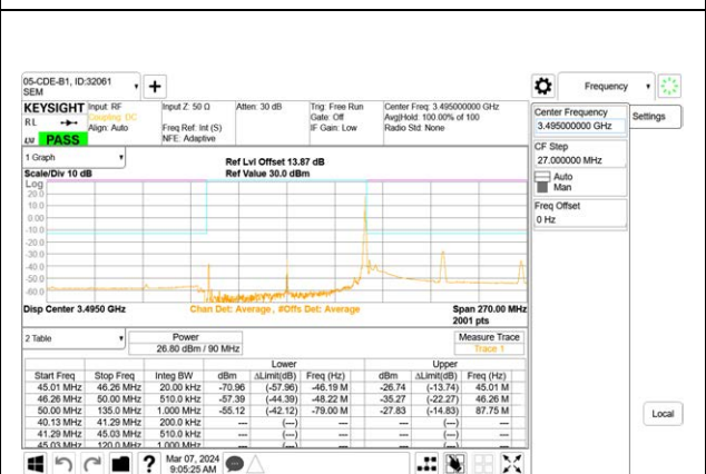
5G NR n77 90MHz BPSK Low Channel RB1-244
