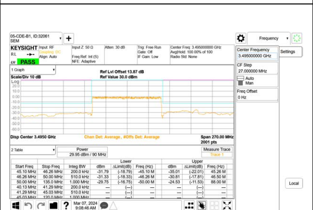
5G NR n77 90MHz BPSK Low Channel RB243-0
