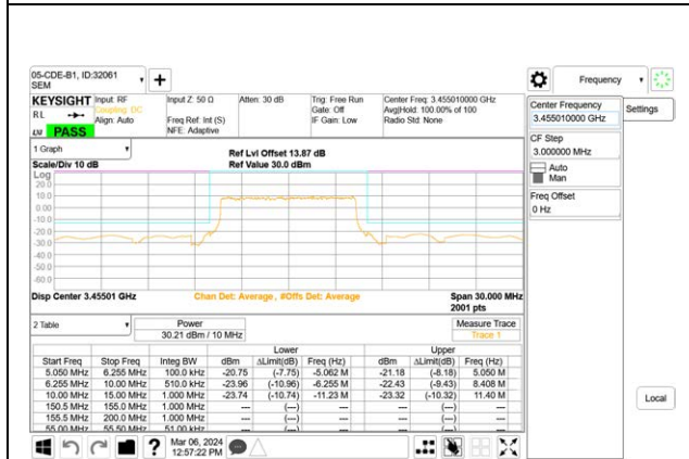
5G NR n77 10MHz BPSK Low Channel RB24-0
