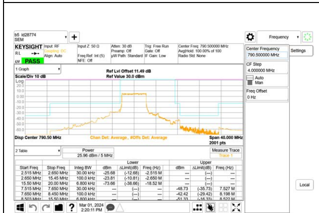
5G NR n14 5MHz BPSK Low Channel RB25-0
