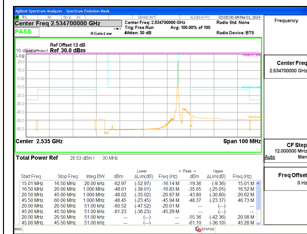
5G NR n7 30MHz BPSK Middle Channel RB1-159, ID:12482
