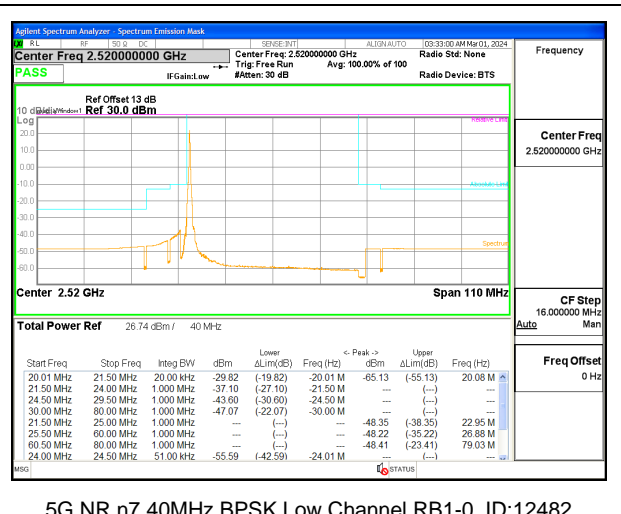
5G NR n7 40MHz BPSK Low Channel RB1-0, ID:12482
