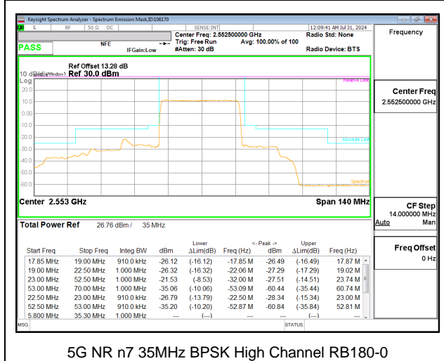
5G NR n7 35MHz BPSK High Channel RB180-0
