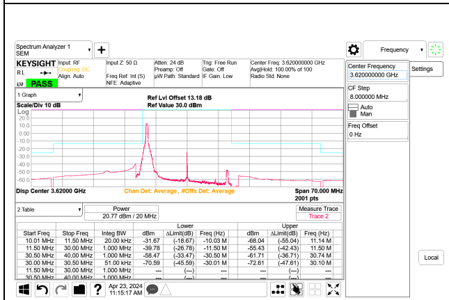
5G NR n48 20MHz QPSK Middle Channel RB1-0 Port B, ID:28567
