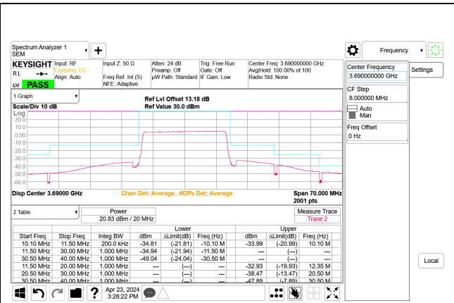
5G NR n48 20MHz QPSK High Channel RB51-0 Port B, ID:28567
