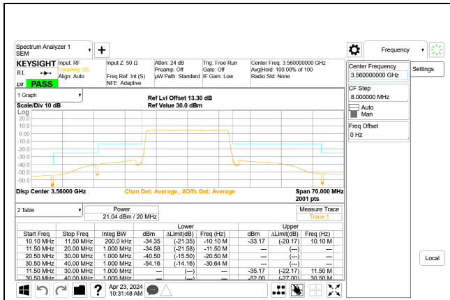
5G NR n48 20MHz QPSK Low Channel RB51-0 Port A, ID:28567
