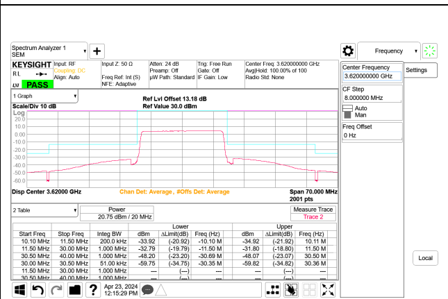
5G NR n48 20MHz QPSK Mid Channel RB51-0 Port B, ID:28567
