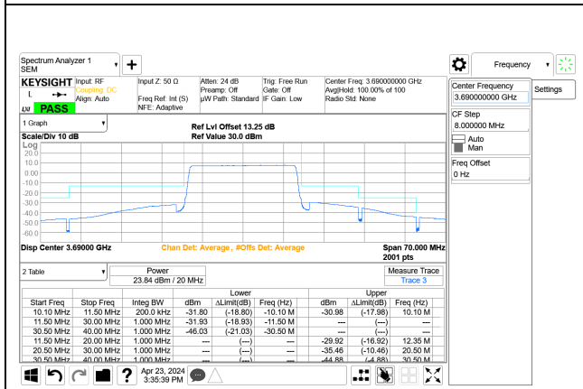
5G NR n48 20MHz QPSK High Channel RB51-0 Port A+B, ID:28567
