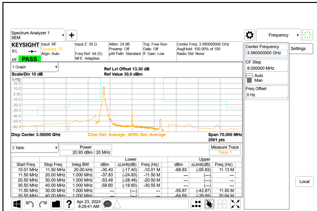
5G NR n48 20MHz QPSK Low Channel RB1-0 Port A, ID:28567
