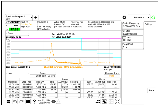
5G NR n48 20MHz QPSK High Channel RB1-0 Port A, ID:28567
