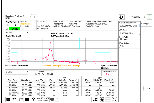
5G NR n48 20MHz QPSK High Channel RB1-0 Port B, ID:28567
