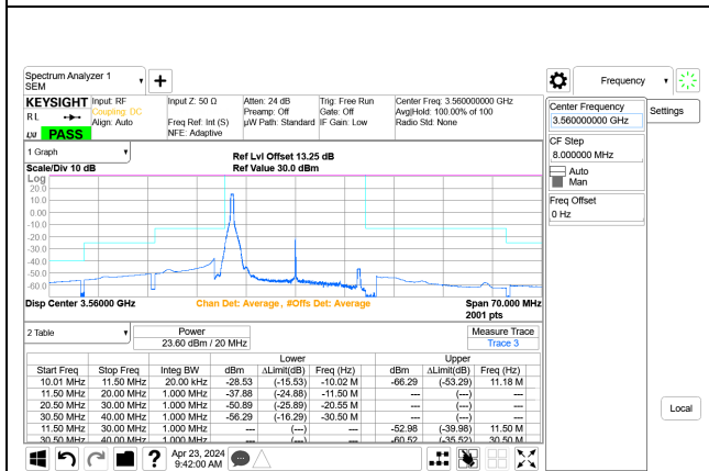
5G NR n48 20MHz QPSK Low Channel RB1-0 Port A+B, ID:28567
