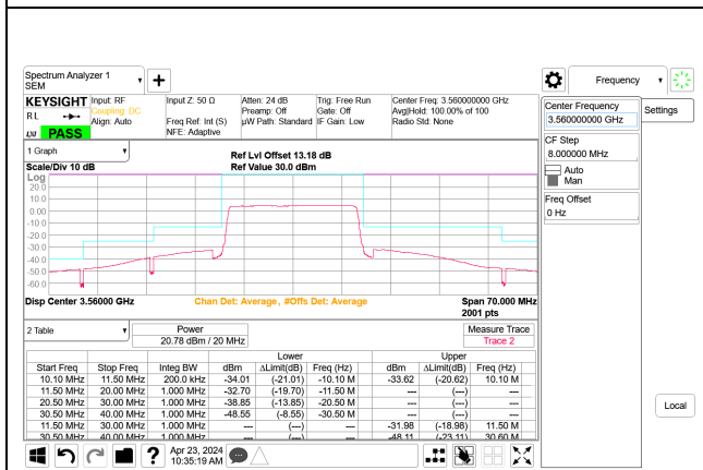
5G NR n48 20MHz QPSK Low Channel RB51-0 Port B, ID:28567
