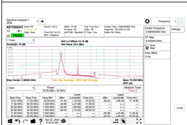
5G NR n48 20MHz QPSK Low Channel RB1-0 Port B, ID:28567
