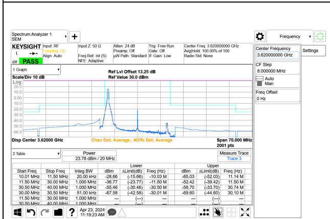
5G NR n48 20MHz QPSK Middle Channel RB1-0 Port A+B, ID:28567
