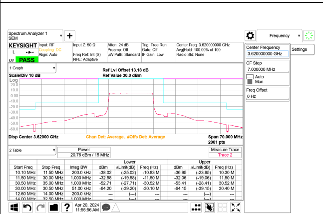
5G NR n48 15MHz QPSK Mid Channel RB38-0 Port B, ID:28567
