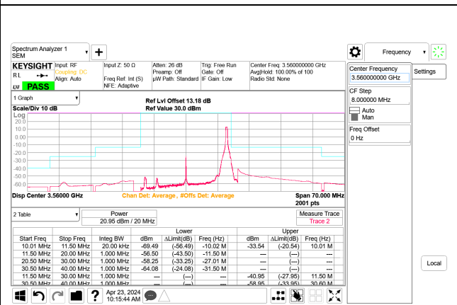
5G NR n48 20MHz QPSK Low Channel RB1-50 Port B, ID:28567
