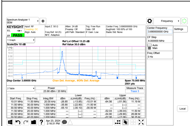
5G NR n48 20MHz QPSK High Channel RB1-0 Port A+B, ID:28567
