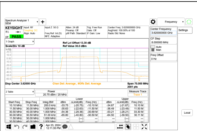
5G NR n48 20MHz QPSK Mid Channel RB51-0 Port A, ID:28567
