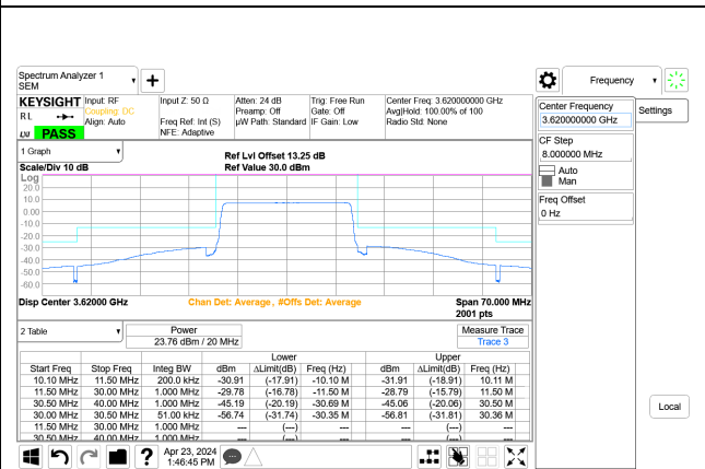
5G NR n48 20MHz QPSK Mid Channel RB51-0 Port A+B, ID:28567
