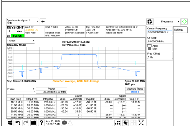
5G NR n48 20MHz QPSK Low Channel RB51-0 Port A+B, ID:28567
