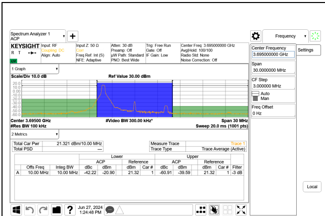
5G NR n48 10MHz QPSK High Channel RB1-0 Port A, ID:32546
