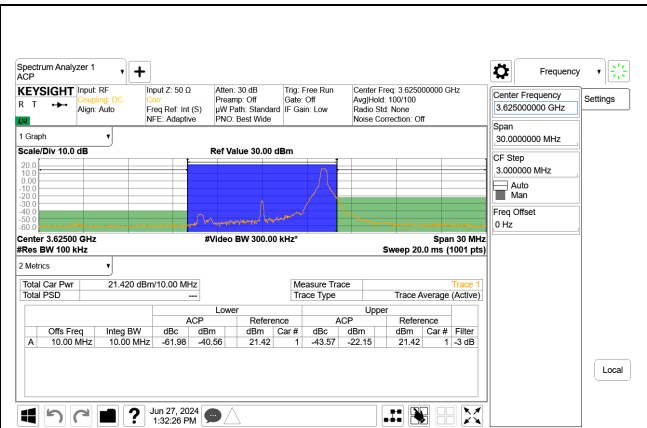
5G NR n48 10MHz QPSK Mid Channel RB1-23 Port A, ID:32546
