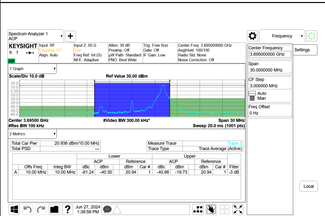
5G NR n48 10MHz QPSK High Channel RB1-23 Port B, ID:32546
