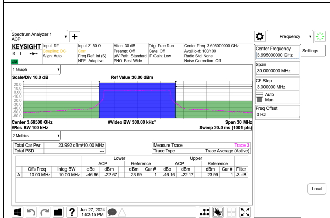
5G NR n48 10MHz QPSK High Channel RB24-0 Port A+B, ID:32546
