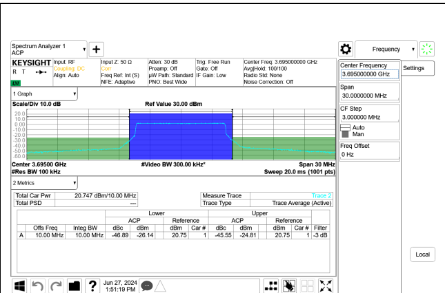
5G NR n48 10MHz QPSK High Channel RB24-0 Port B, ID:32546
