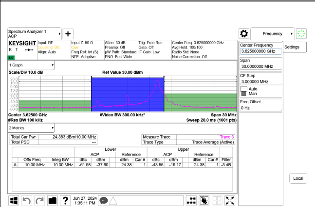
5G NR n48 10MHz QPSK Mid Channel RB1-23 Port A+B, ID:32546
