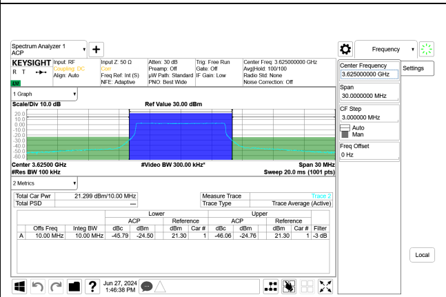
5G NR n48 10MHz QPSK Mid Channel RB24-0 Port B, ID:32546
