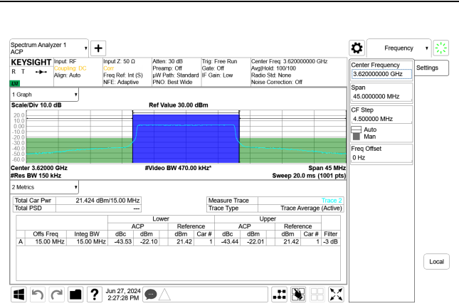
5G NR n48 15MHz BPSK Mid Channel RB38-0 Port B, ID:32546
