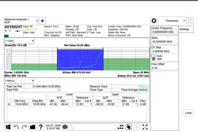
5G NR n48 15MHz BPSK Mid Channel RB1-37 Port B, ID:32546
