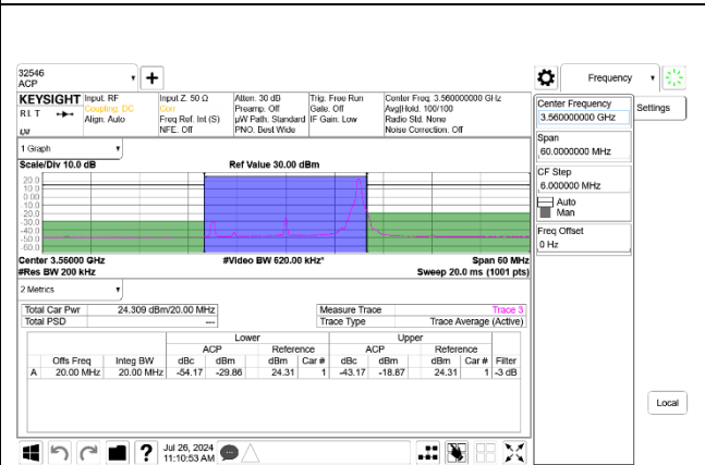
5G NR n48 20MHz BPSK Low Channel RB1-50 Port A+B
