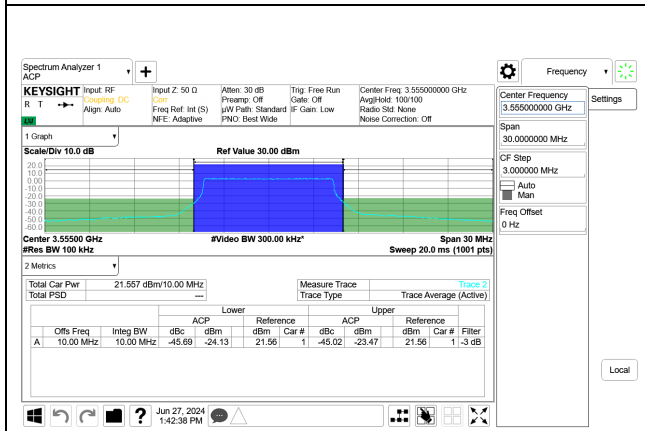
5G NR n48 10MHz QPSK Low Channel RB24-0 Port B, ID:32546
