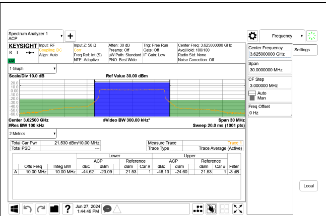
5G NR n48 10MHz QPSK Mid Channel RB24-0 Port A, ID:32546
