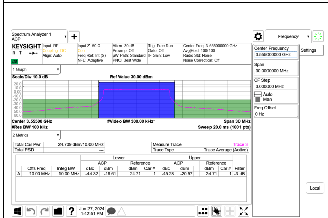
5G NR n48 10MHz QPSK Low Channel RB24-0 Port A+B, ID:32546
