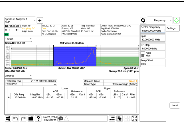
5G NR n48 10MHz QPSK High Channel RB1-23 Port A, ID:32546
