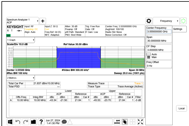
5G NR n48 10MHz QPSK Low Channel RB24-0 Port A, ID:32546
