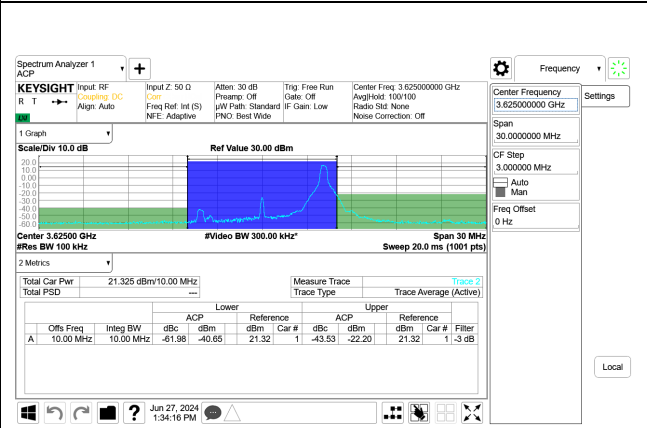
5G NR n48 10MHz QPSK Mid Channel RB1-23 Port B, ID:32546
