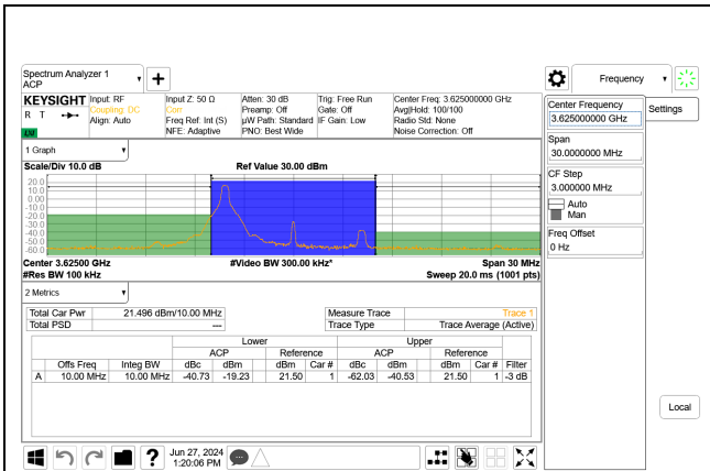
5G NR n48 10MHz QPSK Mid Channel RB1-0 Port A, ID:32546
