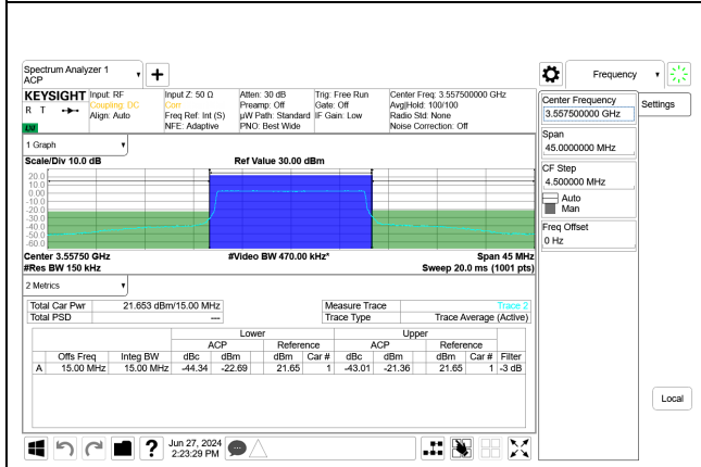
5G NR n48 15MHz BPSK Low Channel RB38-0 Port B, ID:32546
