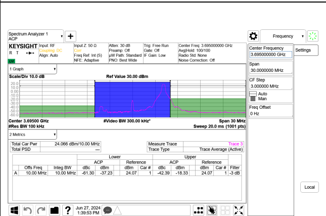
5G NR n48 10MHz QPSK High Channel RB1-23 Port A+B, ID:32546
