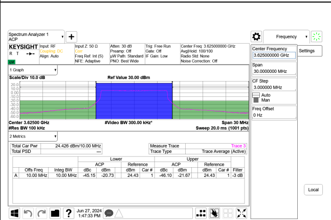
5G NR n48 10MHz QPSK Mid Channel RB24-0 Port A+B, ID:32546
