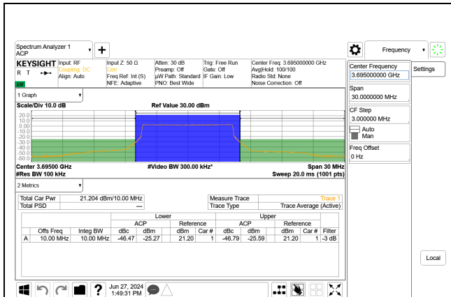
5G NR n48 10MHz QPSK High Channel RB24-0 Port A, ID:32546
