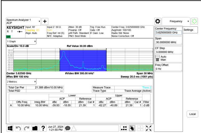
5G NR n48 10MHz QPSK Mid Channel RB1-0 Port B, ID:32546
