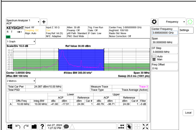
5G NR n48 10MHz QPSK High Channel RB1-0 Port A+B, ID:32546
