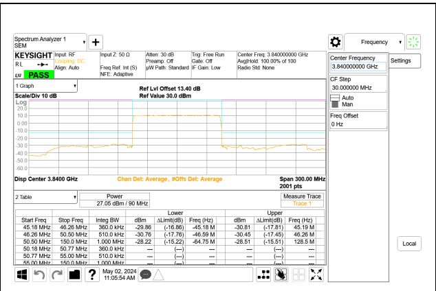
5G NR n77 90MHz BPSK Mid Channel RB243-0 Port A, ID: 32546
