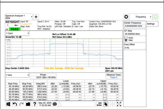
5G NR n77 90MHz BPSK Mid Channel RB243-0 Port A+B, ID: 32546
