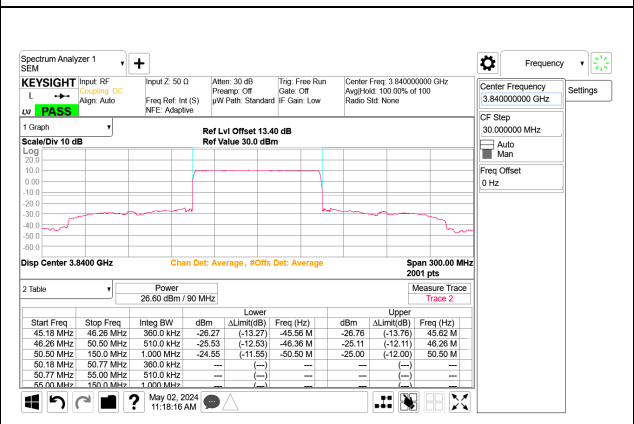
5G NR n77 90MHz BPSK Mid Channel RB243-0 Port B, ID: 32546
