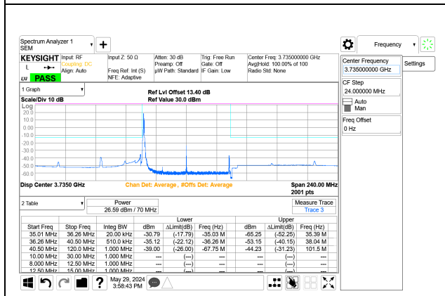
5G NR n77 70MHz BPSK Low Channel RB1-0 Port A+B ID: 32546
