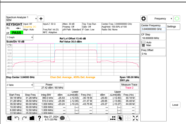
5G NR n77 60MHz BPSK Mid Channel RB162-0 Port B ID: 28774
