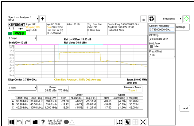
5G NR n77 70MHz BPSK Low Channel RB180-0 Port A ID: 28774
