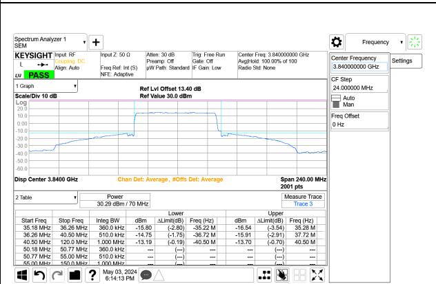
5G NR n77 70MHz BPSK Mid Channel RB180-0 Port A+B, ID: 32546
