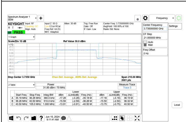
5G NR n77 70MHz BPSK Low Channel RB180-0 Port A+B ID: 28774
