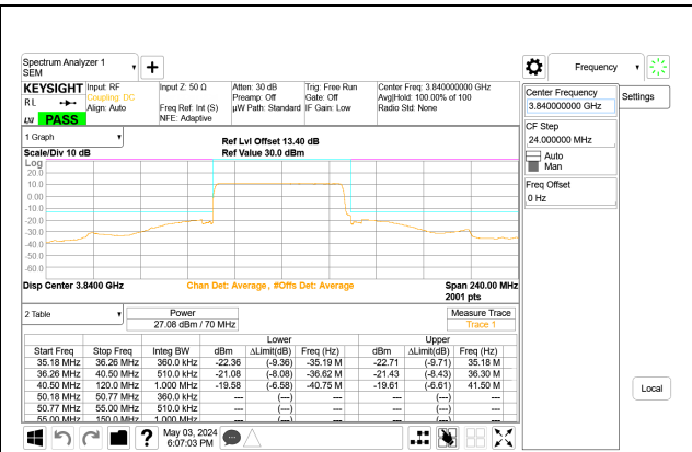
5G NR n77 70MHz BPSK Mid Channel RB180-0 Port A, ID: 32546
