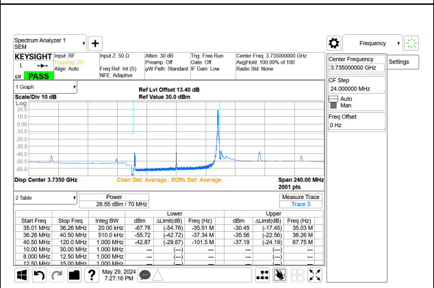
5G NR n77 70MHz BPSK Low Channel RB1-188 Port A+B ID: 32546
