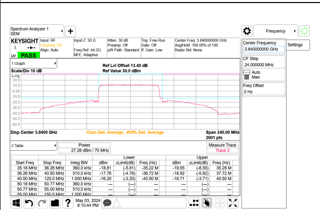
5G NR n77 70MHz BPSK Mid Channel RB180-0 Port B, ID: 32546
